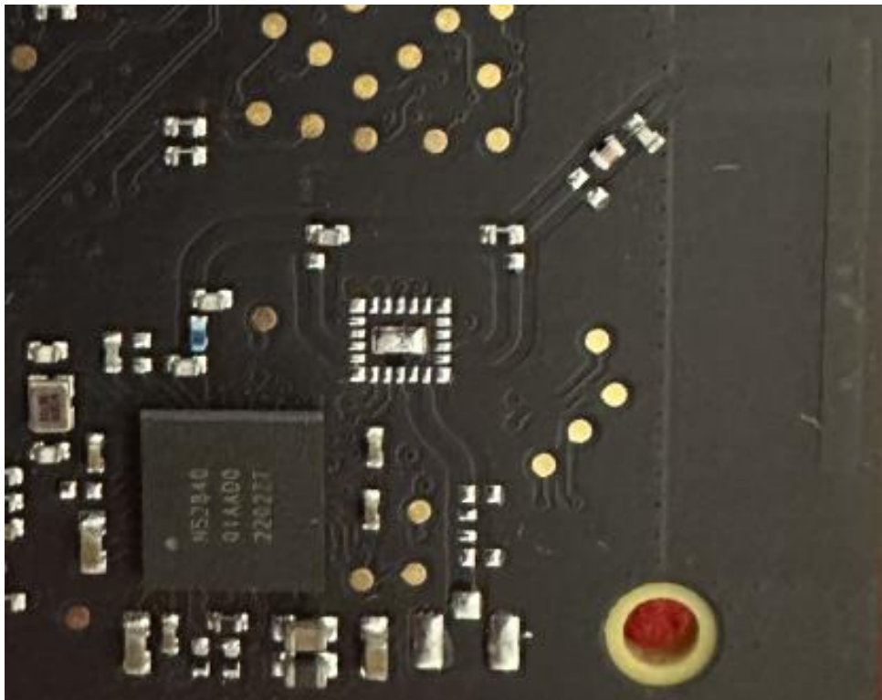
BLE chip
