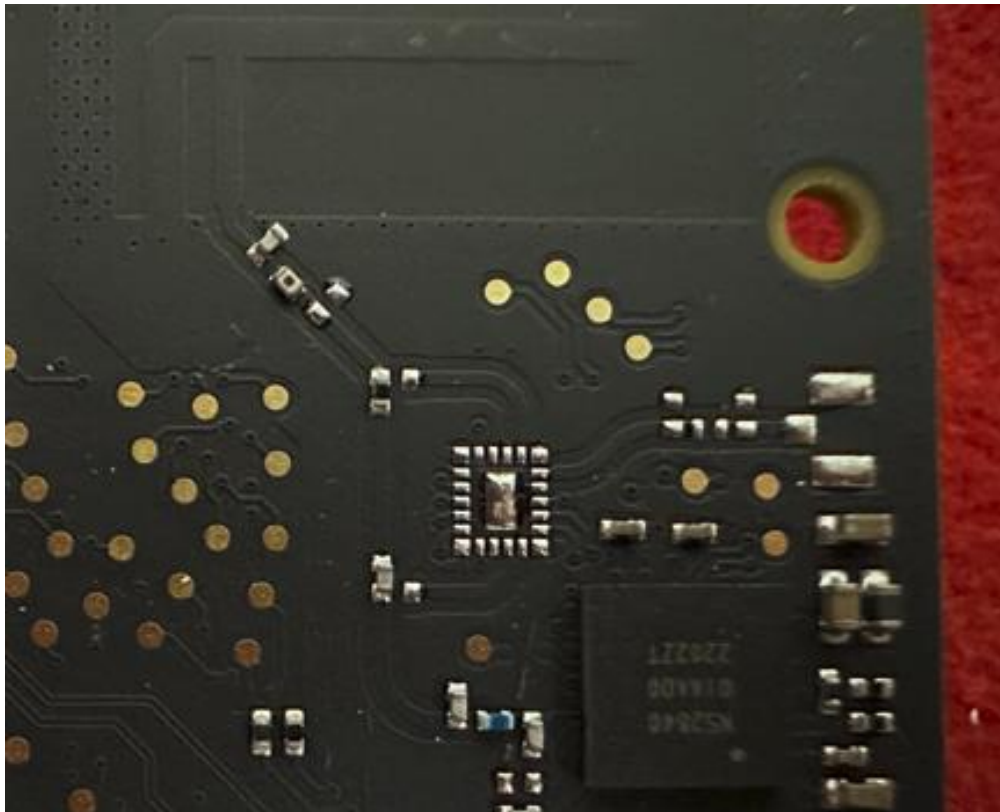
BLE chip
