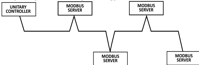
Fig. 33 Modbus Wiring Topology
