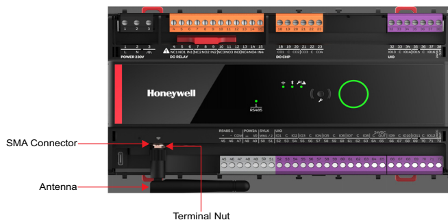
Fig. 28 Antenna
