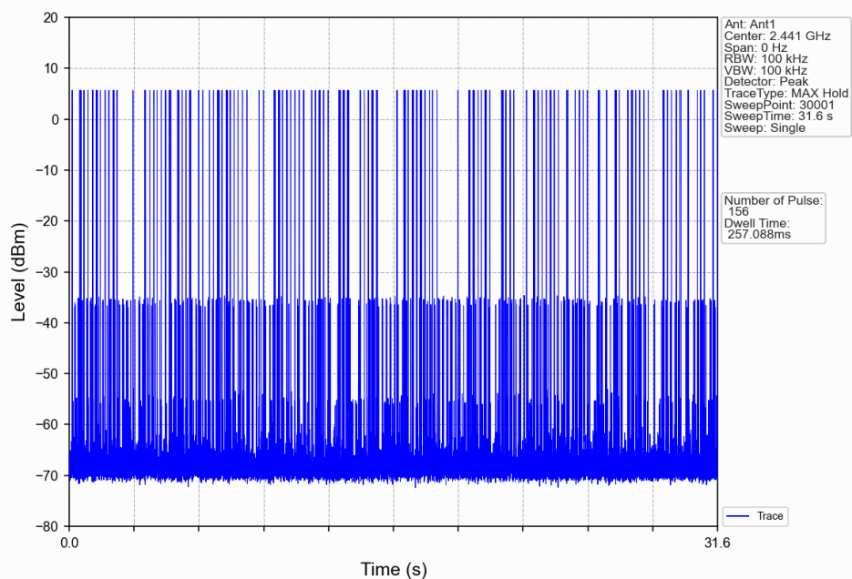
8DPSK 3DH3 HOPP_Ant1_NTNV
