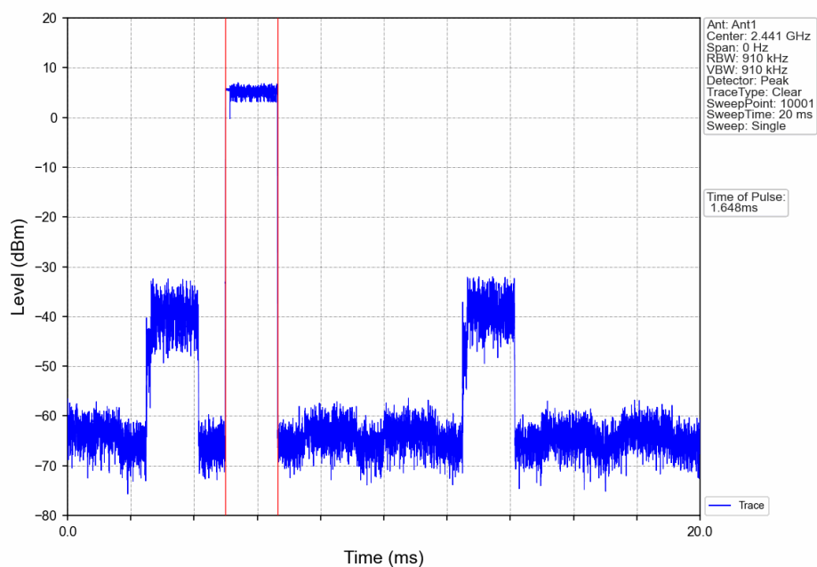
8DPSK 3DH3 HOPP_Ant1_NTNV
