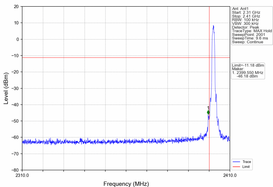
8DPSK 3DH5 LCH 2402MHz Ant1 NTN
