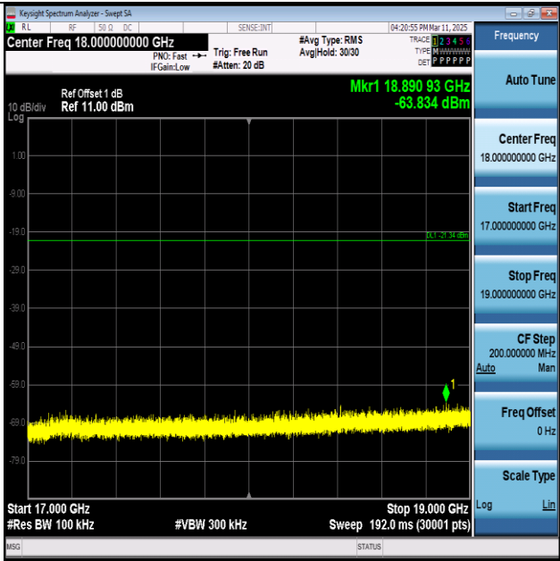
BLE_1M-Ant1-2440-17000~19000-PASS
