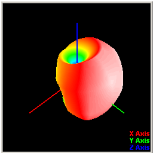
天线方向图
