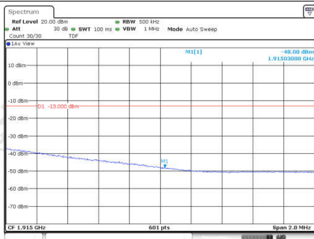
Band25-20MHz-QPSK-26590-1RB#0
