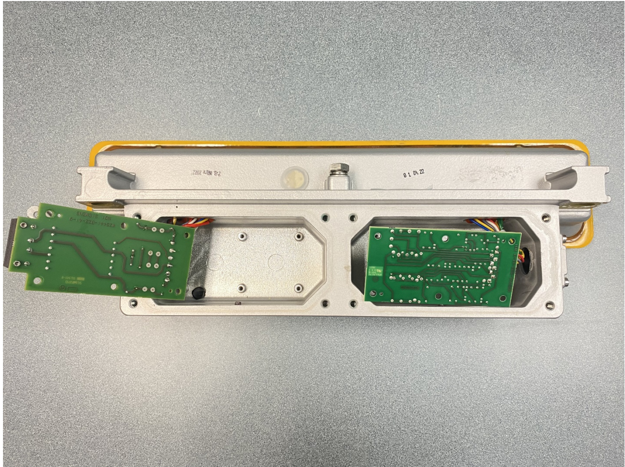
PCB Bottom
