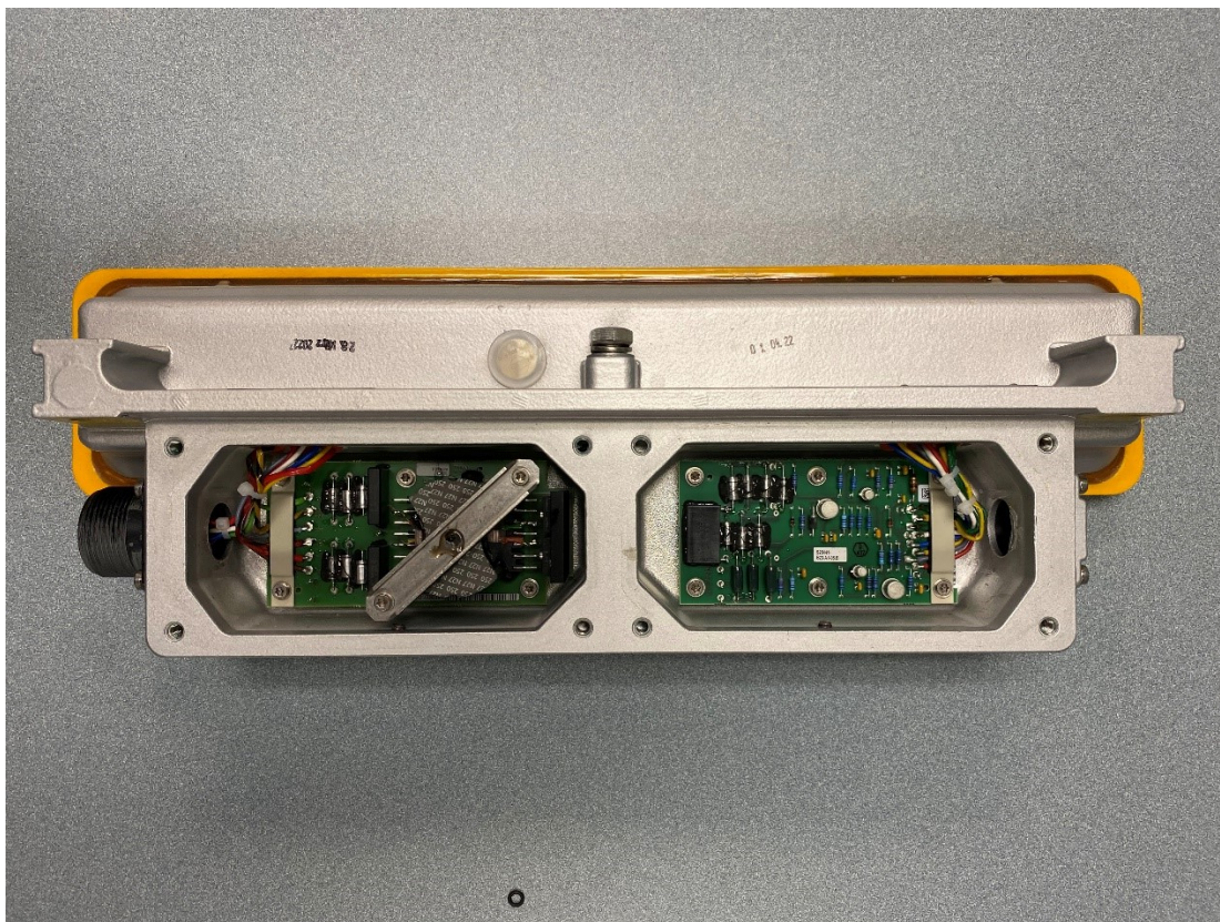
PCB Top
