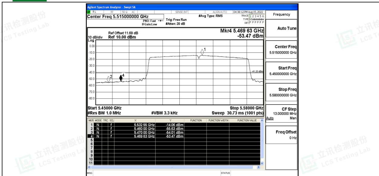
11AC80SISO_Ant0_Low_5530_Peak
