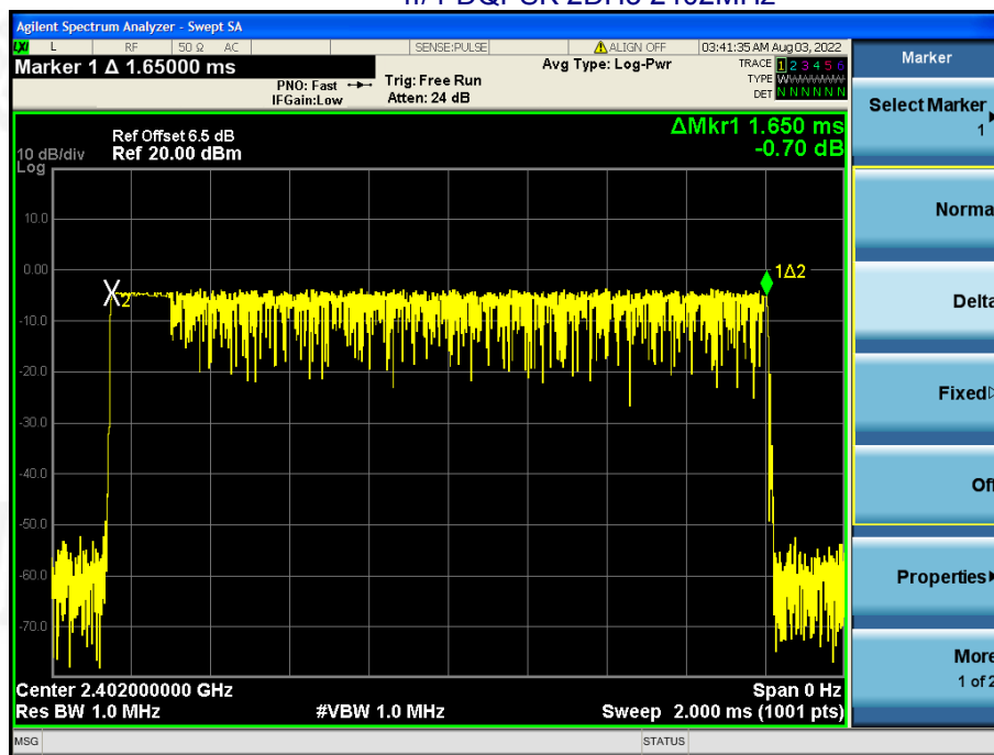
\pi/4 -DQPSK 2DH3 2402MHz
