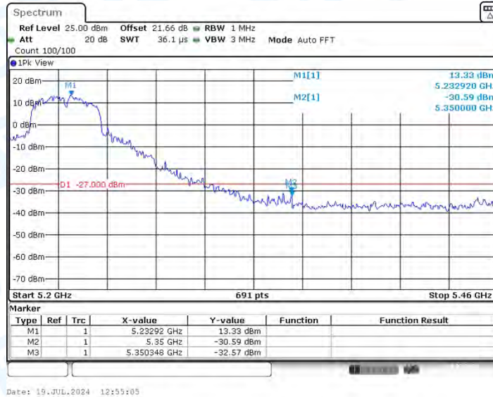
11AC80SISO_Ant1_Low_5210
