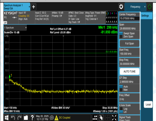
41(2555-2655)-15MHz-QPSK-41165-1RB#0-0.15~30-PASS
