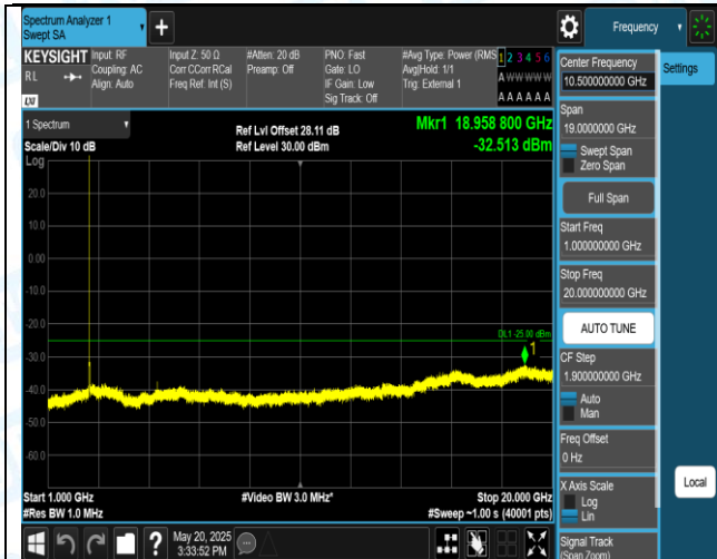
41(2555-2655)-5MHz-16QAM-40265-1RB#0-1000-20000-PASS
