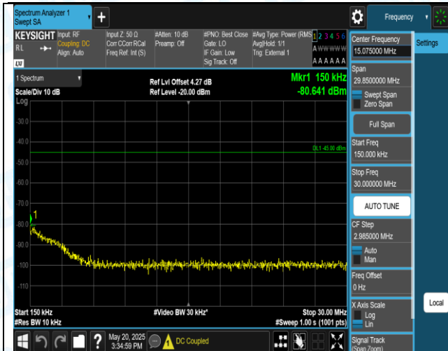
41(2555-2655)-5MHz-QPSK-40690-1RB#0-0.15~30-PASS
