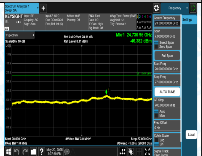
41(2555-2655)-5MHz-QPSK-40690-1RB#0-20000~27000-PASS
