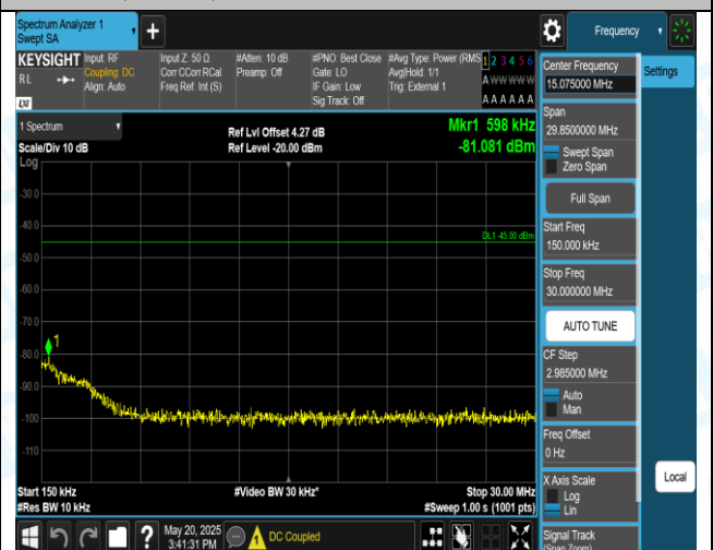
41(2555-2655)-5MHz-QPSK-41215-1RB#0-0.15~30-PASS
