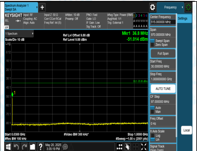
41(2555-2655)-5MHz-QPSK-40690-1RB#0-30~1000-PASS
