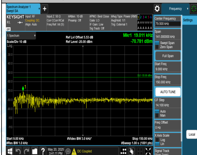
41(2555-2655)-5MHz-QPSK-41215-1RB#0-0.009~0.15-PASS
