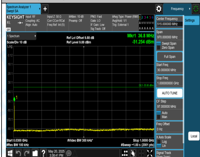
41(2555-2655)-5MHz-16QAM-40690-1RB#0-30-1000-PASS
