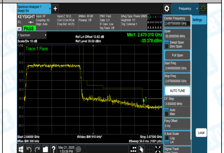
41(2555-2655)-15MHz-QPSK-41165-75RB#0-PASS
