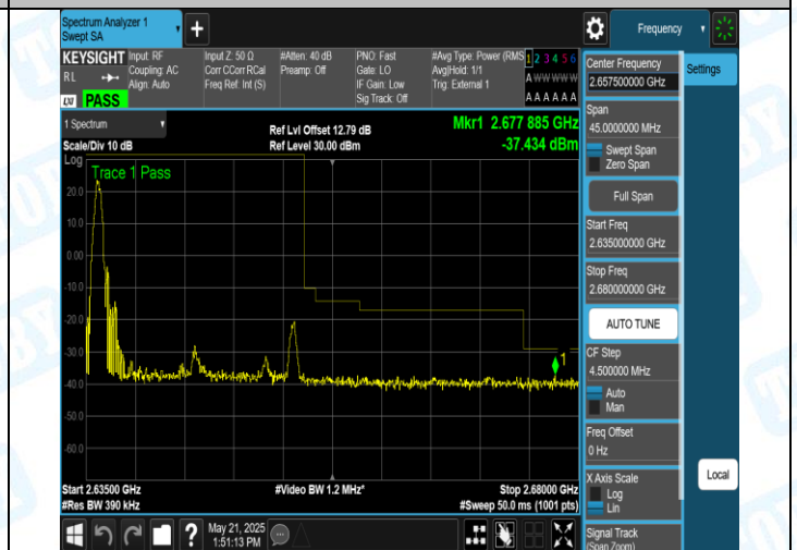
41(2555-2655)-20MHz-16QAM-41140-1RB#0-PASS
