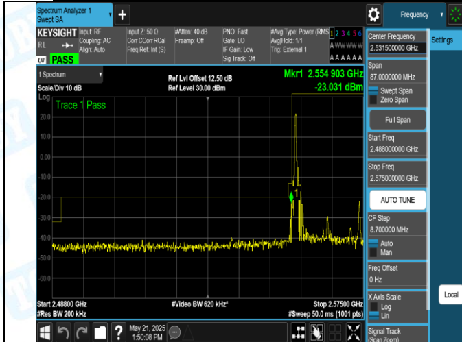
41(2555-2655)-20MHz-16QAM-40340-1RB#0-PASS
