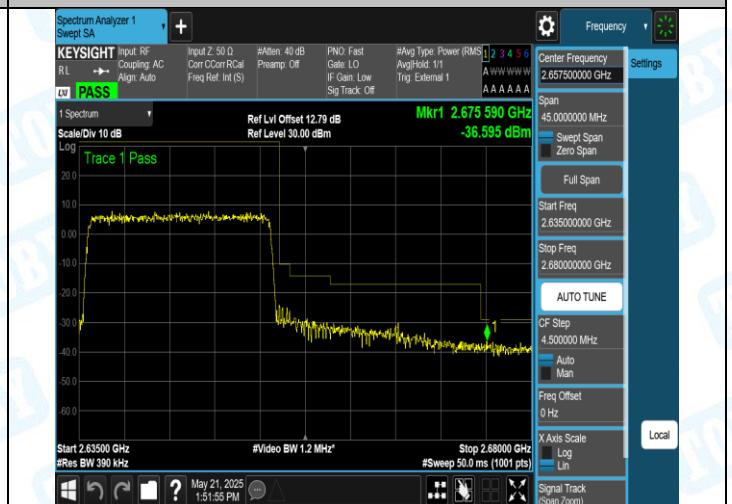
41(2555-2655)-20MHz-16QAM-41140-100RB#0-PASS
