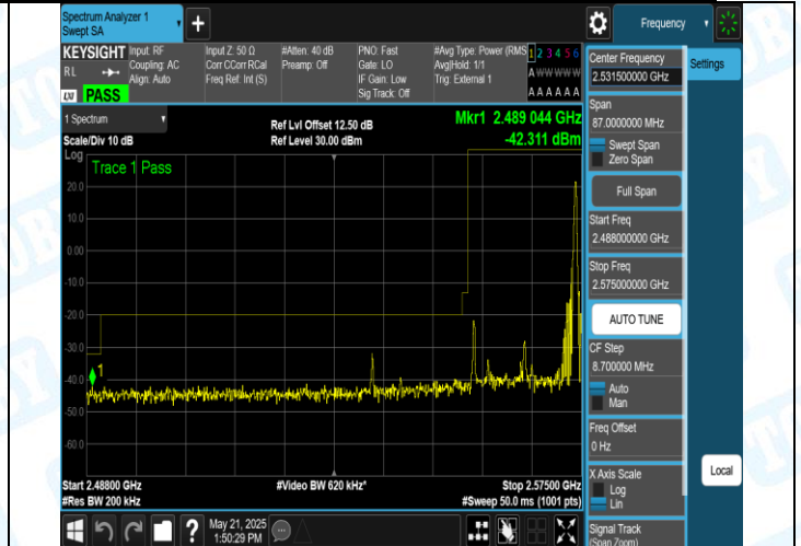
41(2555-2655)-20MHz-16QAM-40340-1RB#99-PASS
