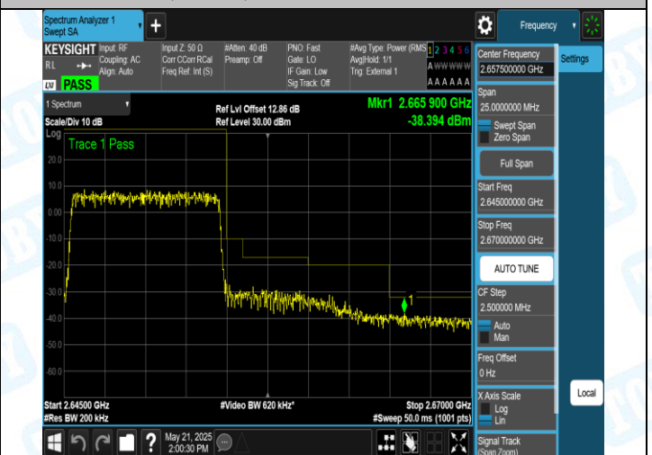
41(2555-2655)-10MHz-16QAM-41190-50RB#0-PASS
