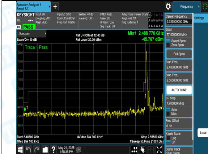
41(2555-2655)-10MHz-QPSK-40290-1RB#0-PASS
