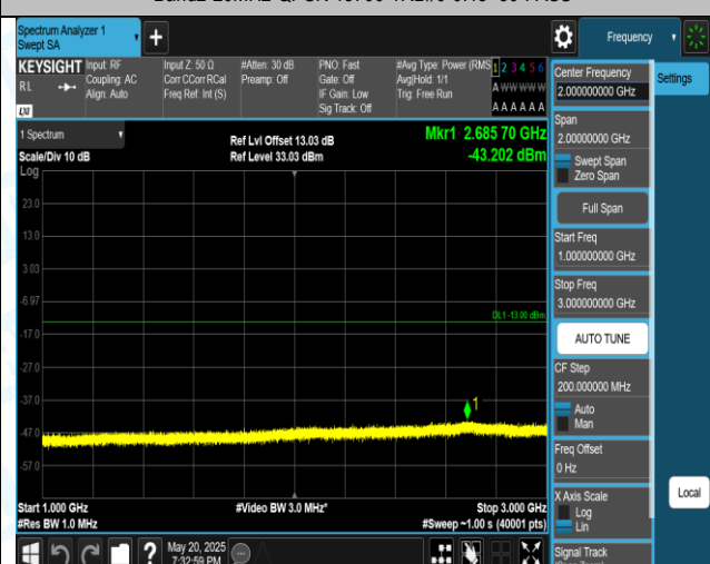
Band2-20MHz-QPSK-18700-1RB#0-1000~3000-PASS
