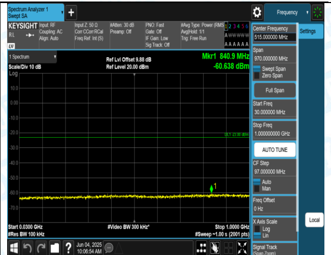
Band2-10MHz-QPSK-18900-1RB#0-30-1000-PASS
