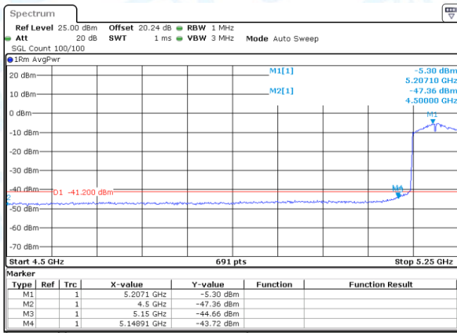
11AC80SISO-Ant1-5210-PASS
