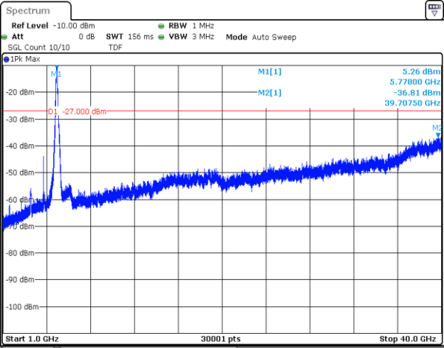
11AC80SISO-Ant1-5775-1000~40000-PASS
