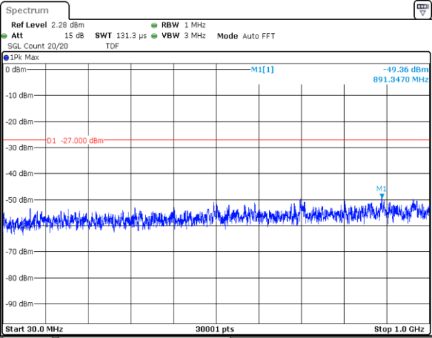
11AC80SISO-Ant1-5775-30~1000-PASS
