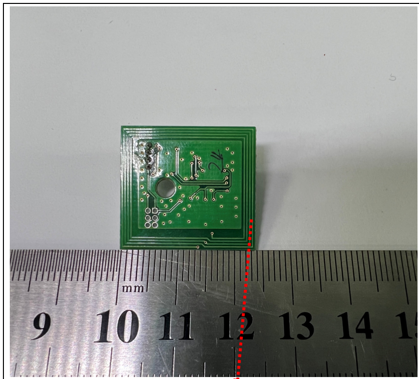
<NFC Antenna>
