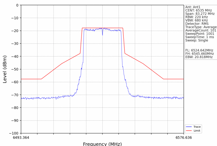
802.11ax(HEW20)_LCH_6535MHz_RU242_Left_Ant1_NTNV
