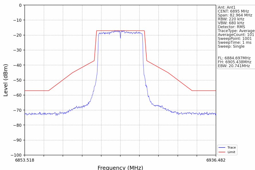
802.11ax(HEW20)_LCH_6895MHz_RU242_Left_Ant1_NTNV
