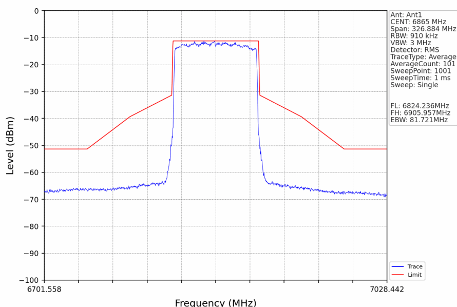
802.11ax(HEW80)_HCH_6865MHz_RU996_Left_Ant1_NTNV
