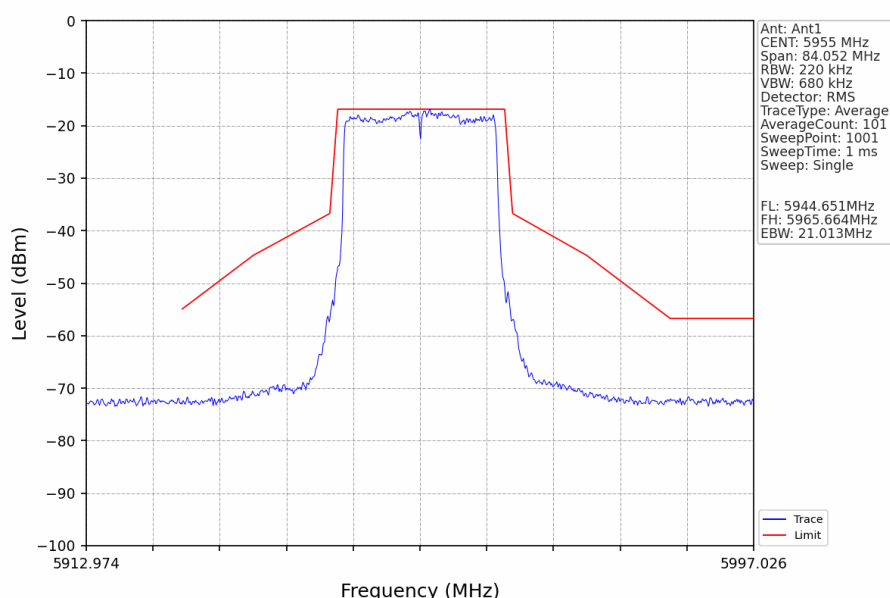
802.11ax(HEW20)_LCH_5955MHz_RU242_Left_Ant1_NTNV
