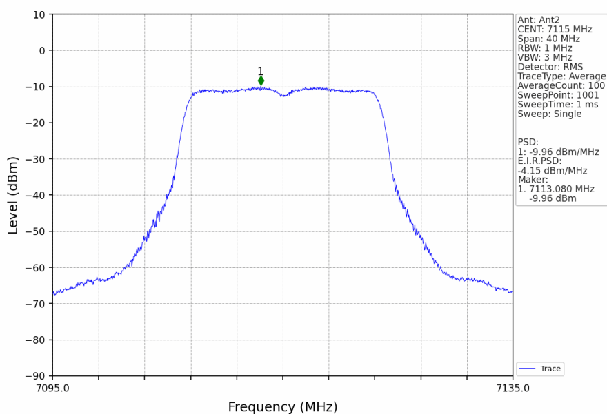
802.11a_HCH_7115MHz_Ant2_NTNV
