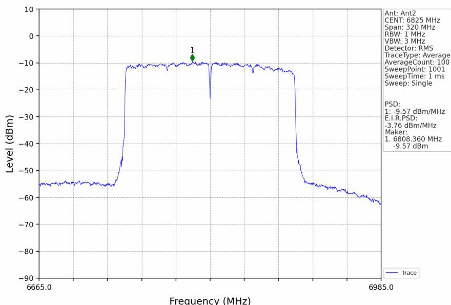
802.11ax(HEW160)_HCH_6825MHz_2xRU996_Left_Ant2_NTNV
