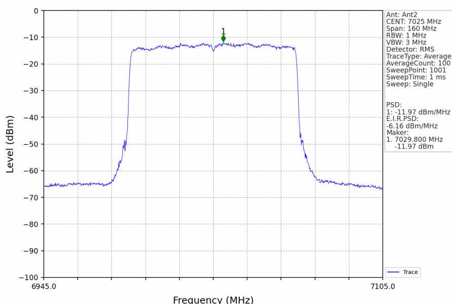
802.11ax(HEW80)_HCH_7025MHz_RU996_Left_Ant2_NTNV
