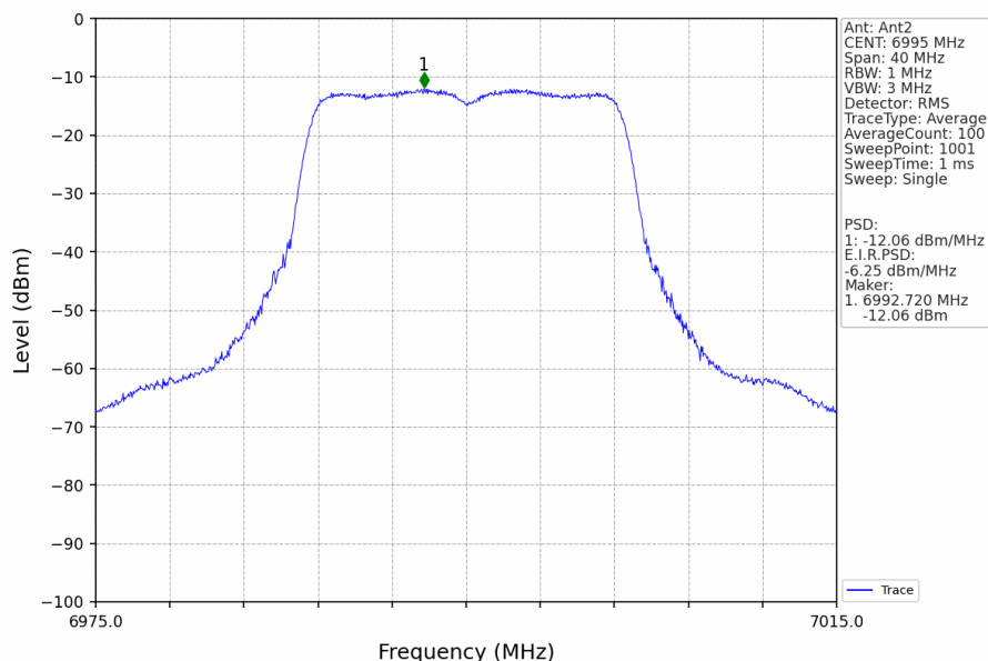
802.11a_MCH_6995MHz_MIMO_NTNV
