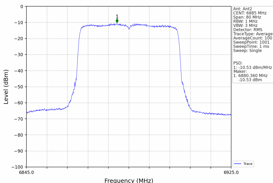
802.11ax(HEW40)_HCH_6885MHz_RU484_Left_Ant2_NTNV
