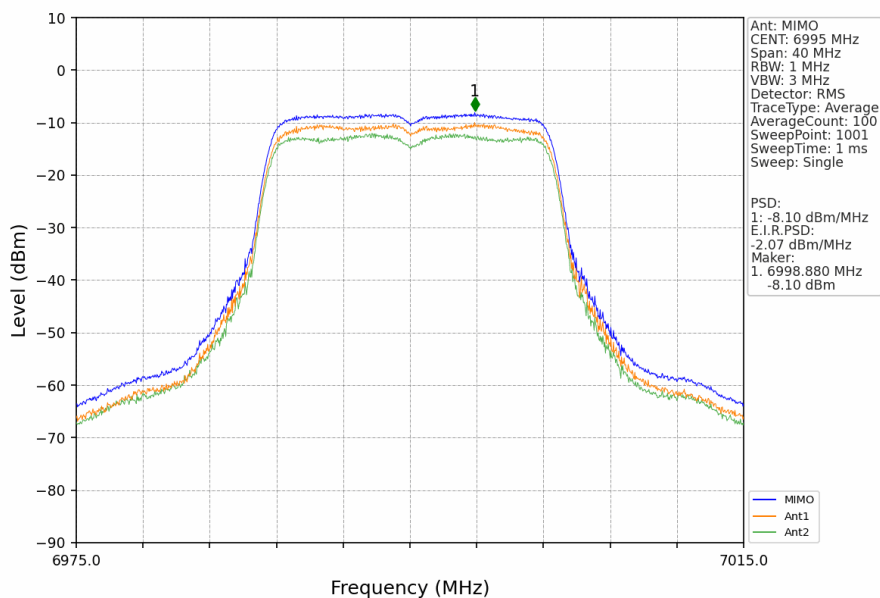
802.11a_MCH_6995MHz_MIMO_NTNV
