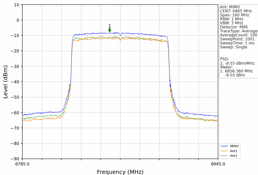
802.11ax(HEW80)_HCH_6865MHz_RU996_Left_MIMO_NTNV
