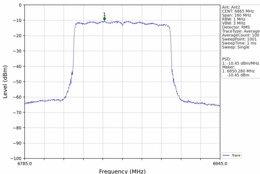
802.11ax(HEW80)_HCH_6865MHz_RU996_Left_MIMO_NTNV
