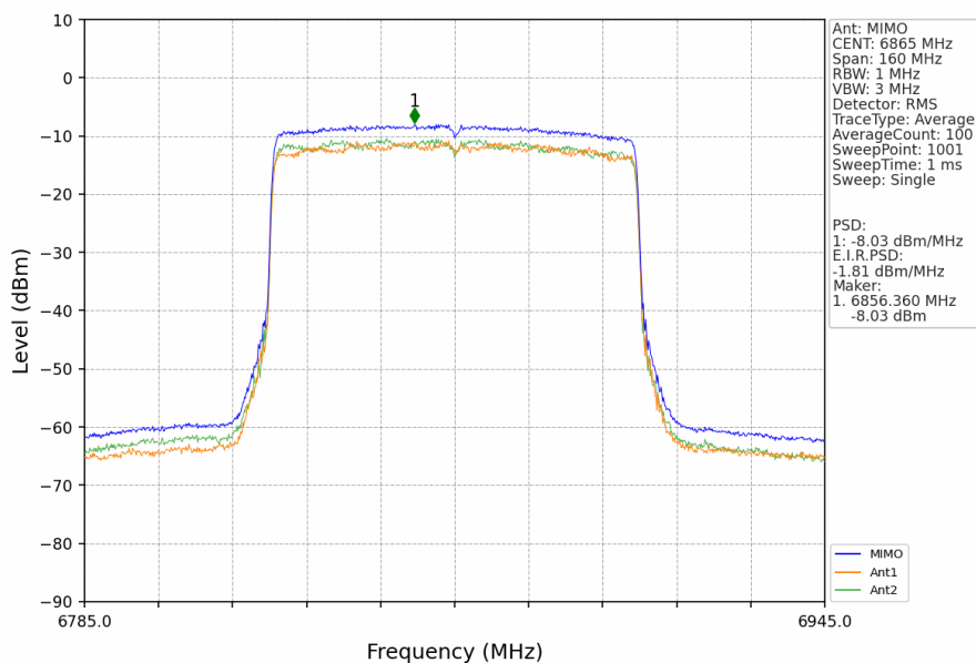
802.11ax(HEW80)_HCH_6865MHz_RU996_Left_MIMO_NTNV
