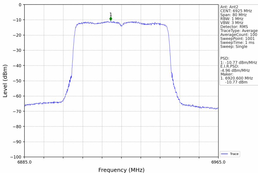
802.11ax(HEW40)_LCH_6925MHz_RU484_Left_Ant2_NTNV
