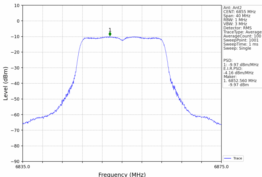
802.11a_HCH_6855MHz_Ant2_NTNV
