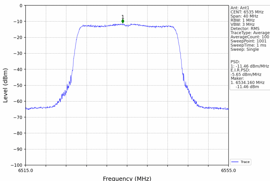
802.11ax(HEW20)_LCH_6535MHz_RU242_Left_Ant1_NTNV
