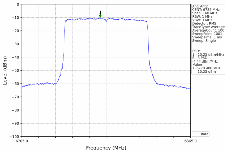
802.11ax(HEW80)_HCH_6785MHz_RU996_Left_MIMO_NTNV
