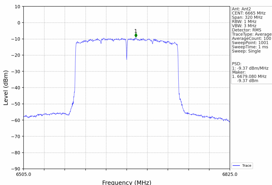
802.11ax(HEW160)_MCH_6665MHz_2xRU996_Left_Ant2_NTNV
