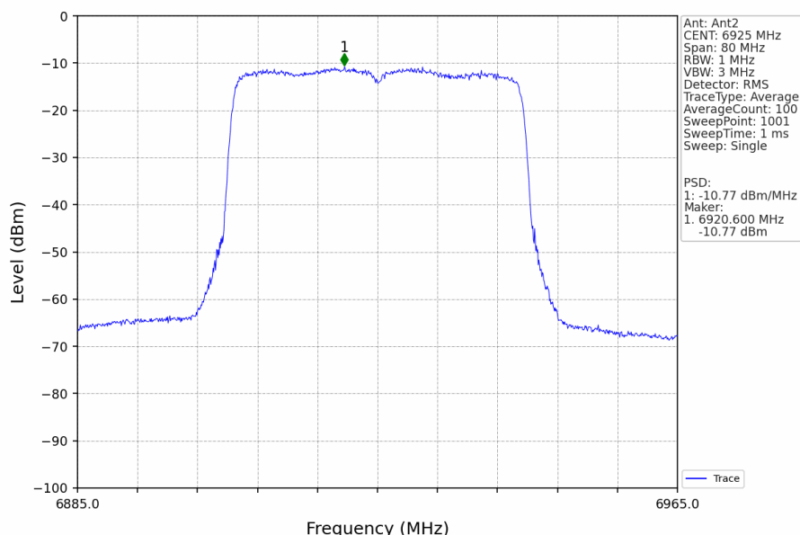
802.11ax(HEW40)_LCH_6925MHz_RU484_Left_Ant2_NTNV
