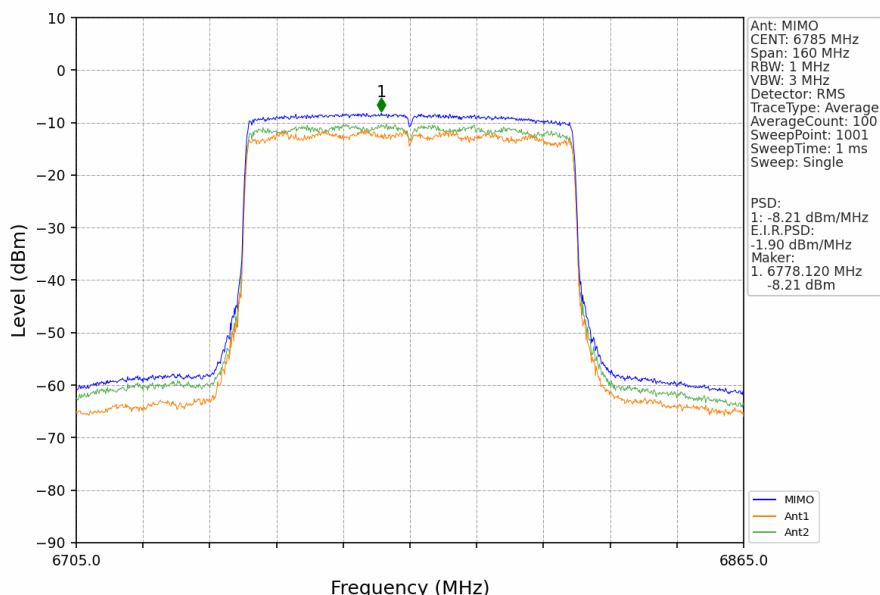
802.11ax(HEW80)_HCH_6785MHz_RU996_Left_MIMO_NTNV
