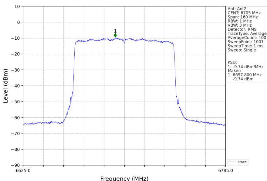
802.11ax(HEW80)_MCH_6705MHz_RU996_Left_Ant2_NTNV
