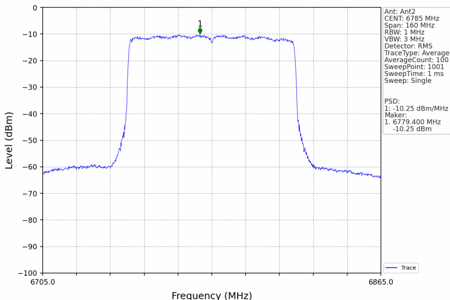
802.11ax(HEW80)_HCH_6785MHz_RU996_Left_MIMO_NTNV
