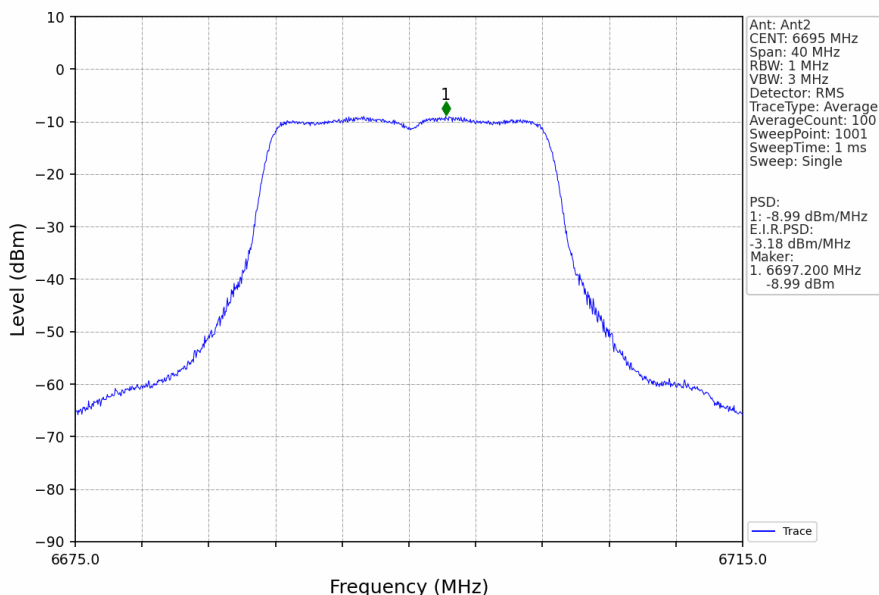
802.11a_MCH_6695MHz_MIMO_NTNV
