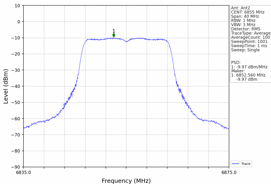
802.11a_HCH_6855MHz_Ant2_NTNV
