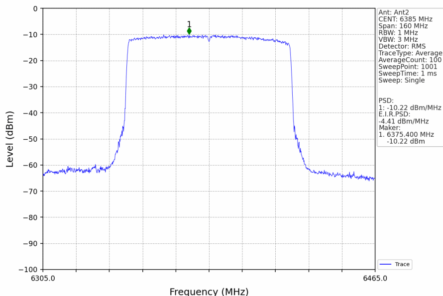
802.11ax(HEW80)_HCH_6385MHz_RU996_Left_MIMO_NTNV
