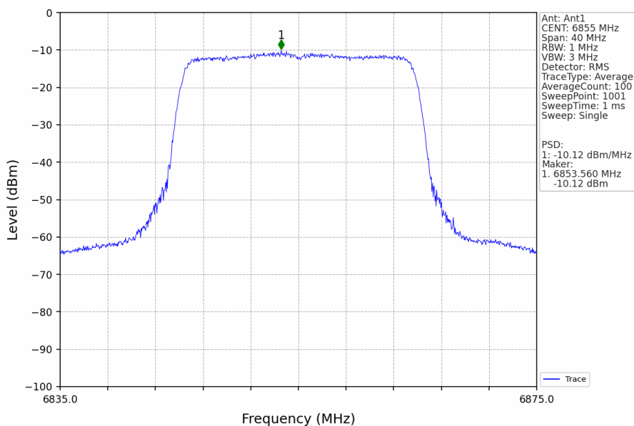
802.11ax(HEW20)_HCH_6855MHz_RU242_Left_Ant1_NTNV
