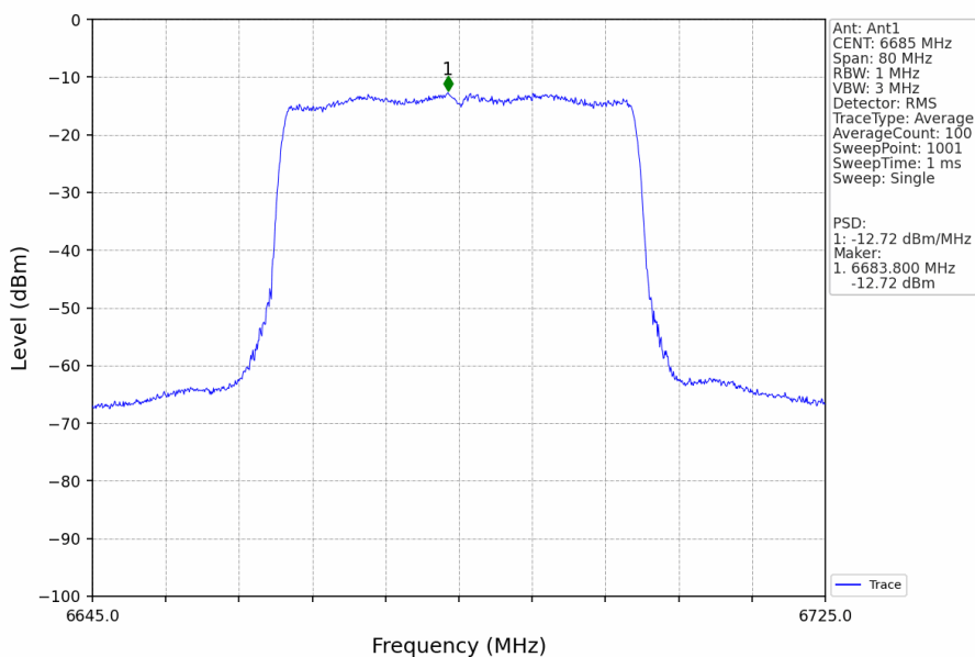
802.11ax(HEW40)_MCH_6685MHz_RU484_Left_Ant1_NTNV
