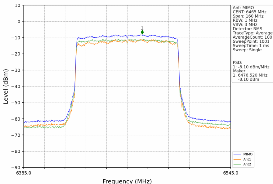
802.11ax(HEW80)_LCH_6465MHz_RU996_Left_MIMO_NTNV
