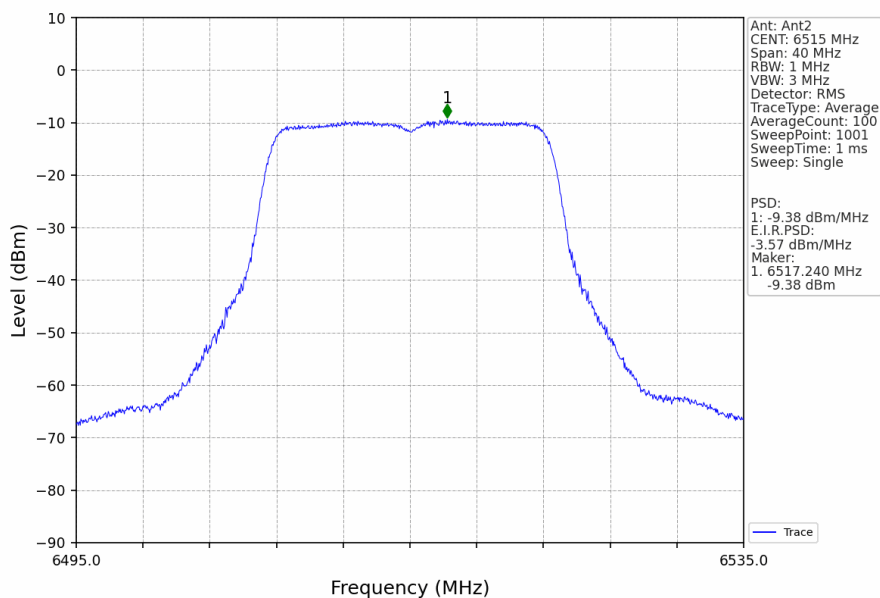
802.11a_HCH_6515MHz_Ant2_NTNV
