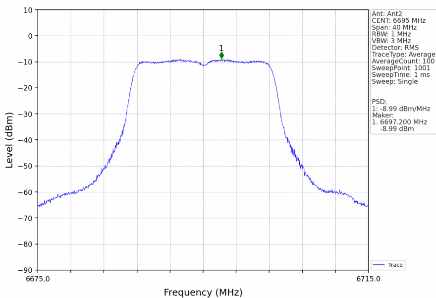
802.11a_MCH_6695MHz_MIMO_NTNV
