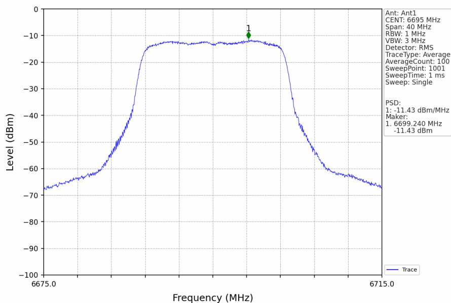
802.11a_MCH_6695MHz_Ant1_NTNV
