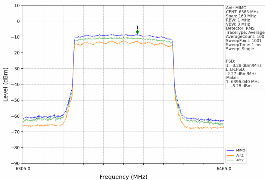
802.11ax(HEW80)_HCH_6385MHz_RU996_Left_MIMO_NTNV
