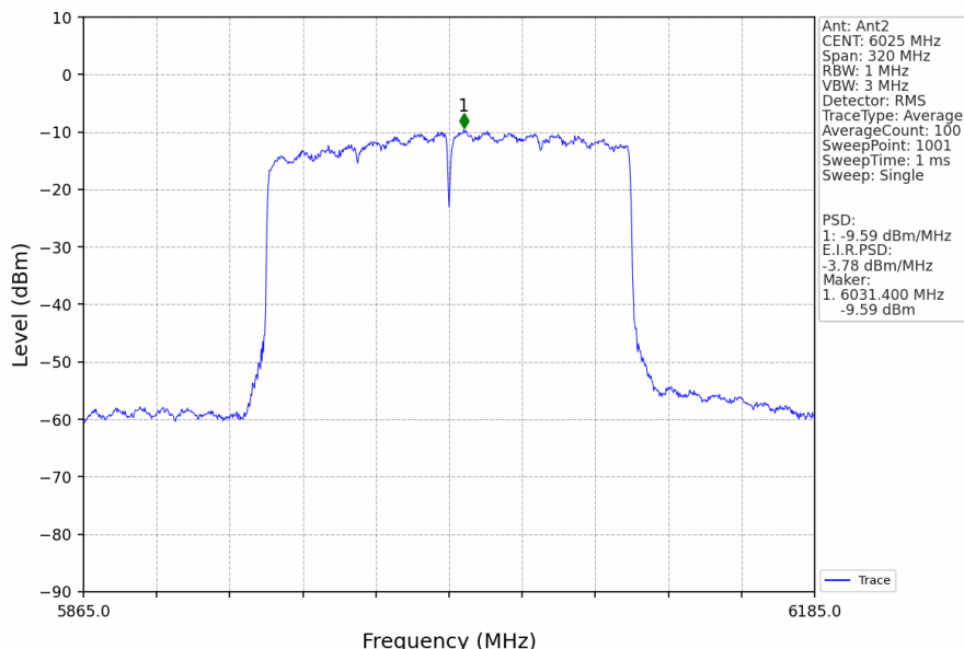
802.11ax(HEW160)_LCH_6025MHz_2xRU996_Left_Ant2_NTNV
