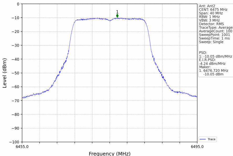
802.11a_MCH_6475MHz_MIMO_NTNV
