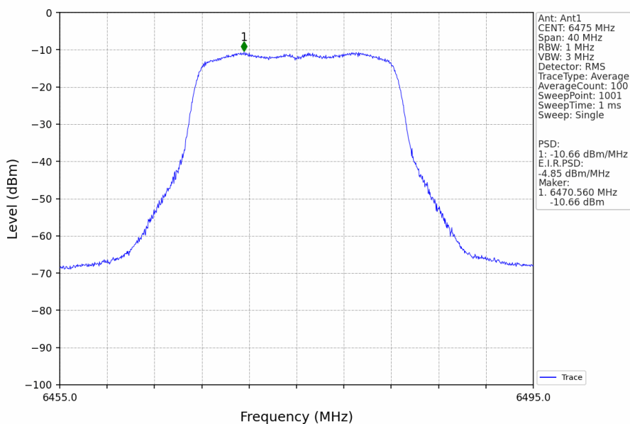
802.11a_MCH_6475MHz_Ant1_NTNV
