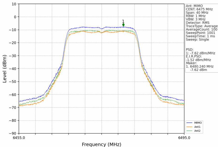
802.11a_MCH_6475MHz_MIMO_NTNV
