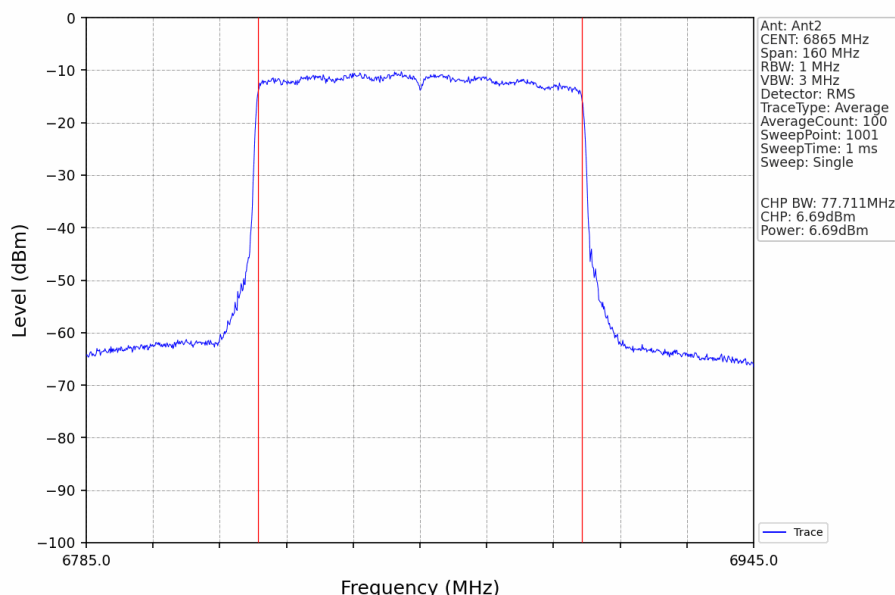
802.11ax(HEW80)_HCH_6865MHz_RU996_Left_Ant2_NTNV
