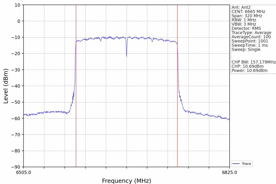
802.11ax(HEW160)_MCH_6665MHz_2xRU996_Left_Ant2_NTNV
