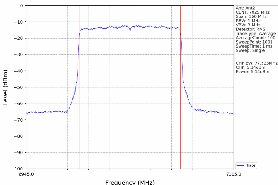
802.11ax(HEW80)_HCH_7025MHz_RU996_Left_Ant2_NTNV
