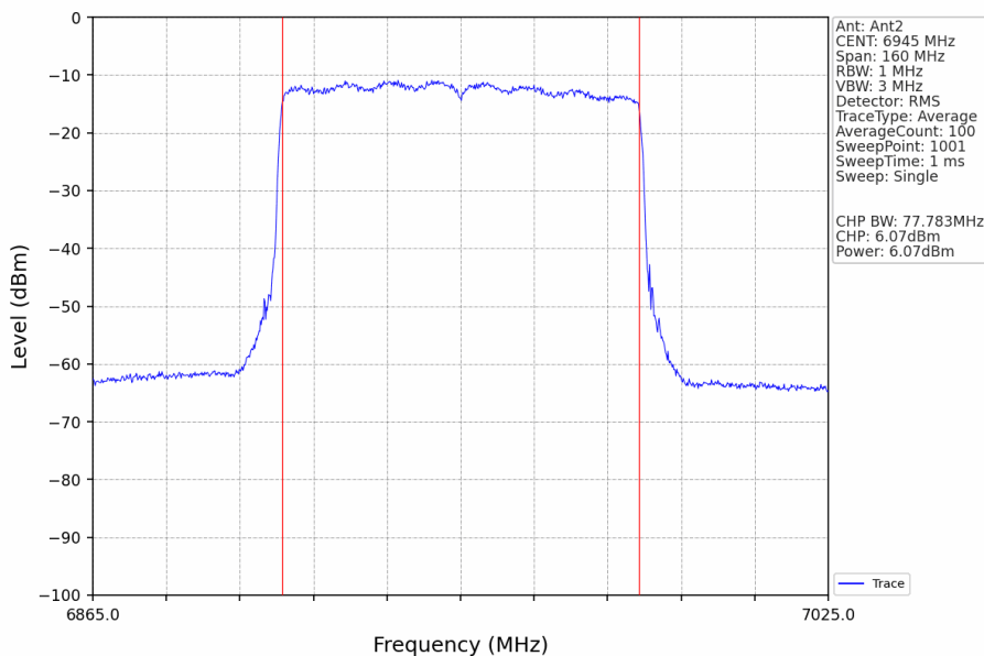
802.11ax(HEW80)_LCH_6945MHz_RU996_Left_Ant2_NTNV
