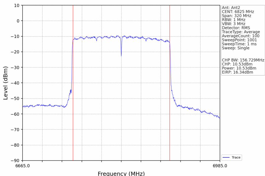
802.11ax(HEW160)_HCH_6825MHz_2xRU996_Left_Ant2_NTNV
