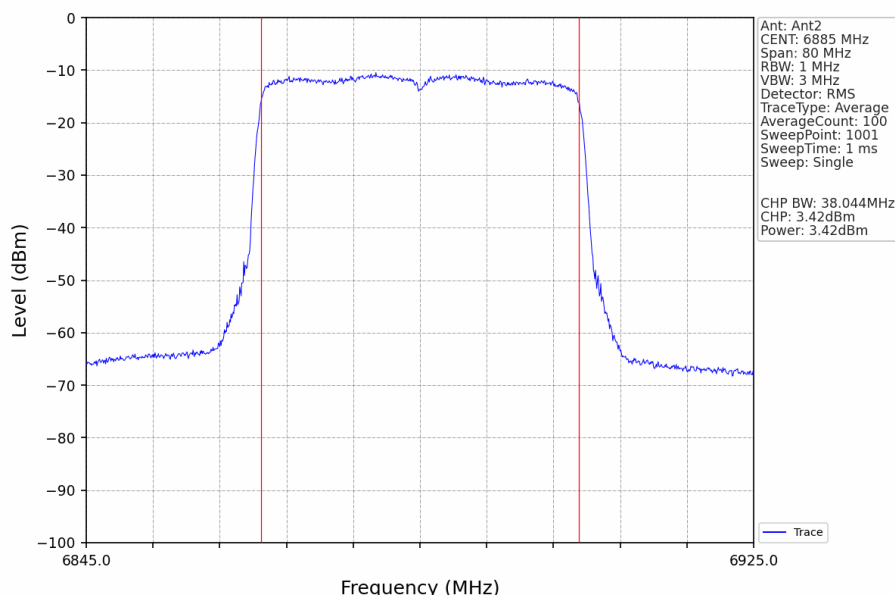
802.11ax(HEW40)_HCH_6885MHz_RU484_Left_Ant2_NTNV
