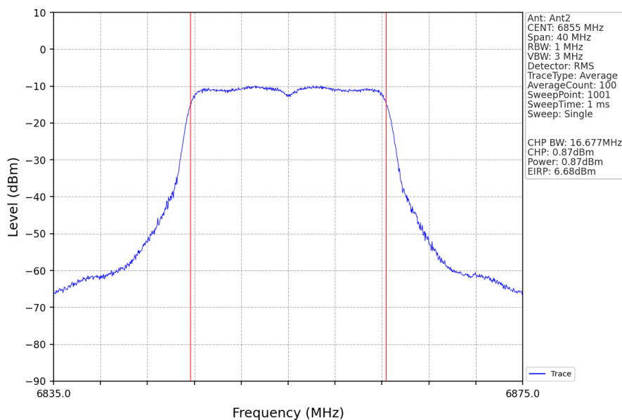
802.11a_HCH_6855MHz_Ant2_NTNV
