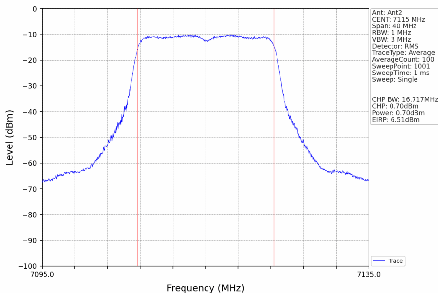
802.11a_HCH_7115MHz_Ant2_NTNV
