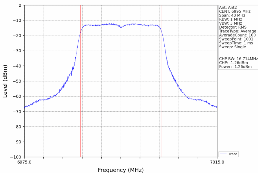
802.11a_MCH_6995MHz_Ant2_NTNV
