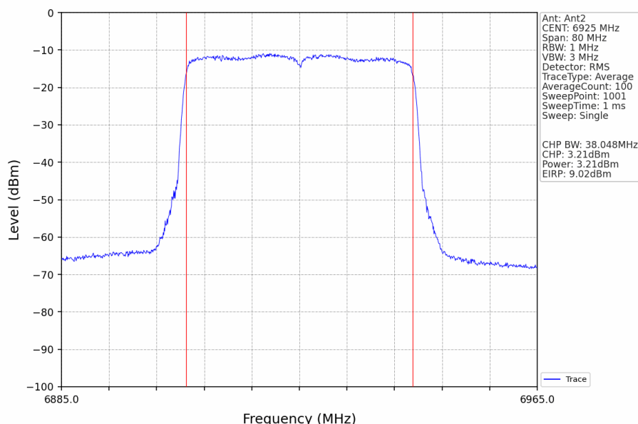
802.11ax(HEW40)_LCH_6925MHz_RU484_Left_Ant2_NTNV
