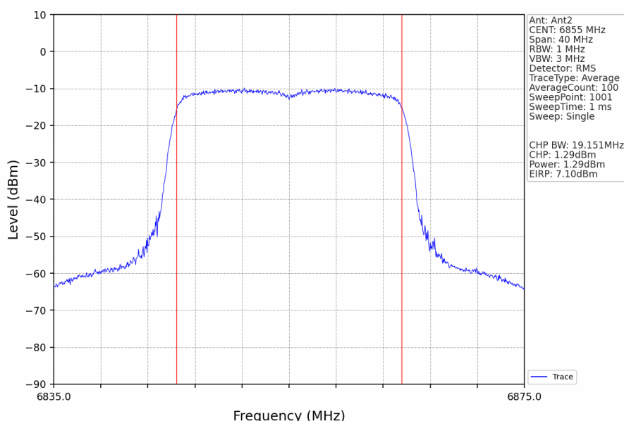
802.11ax(HEW20)_HCH_6855MHz_RU242_Left_Ant2_NTNV
