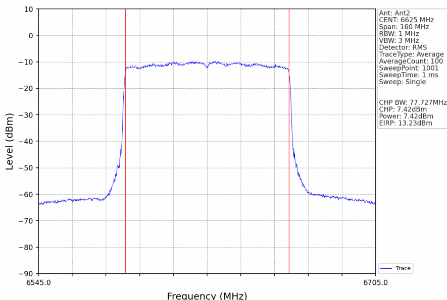
802.11ax(HEW80)_LCH_6625MHz_RU996_Left_Ant2_NTNV
