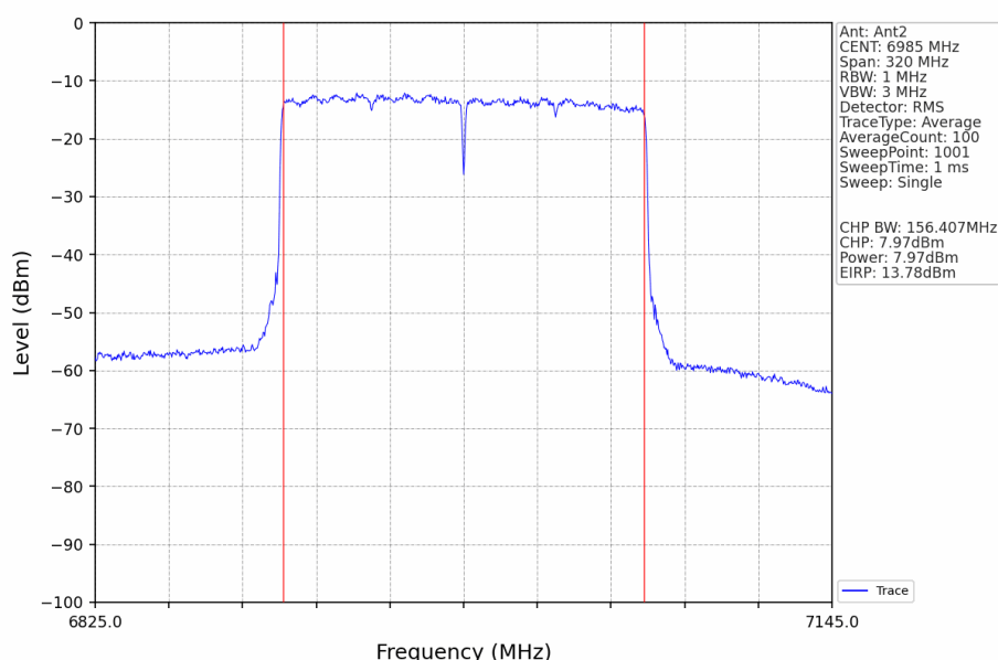
802.11ax(HEW160)_MCH_6985MHz_2xRU996_Left_Ant2_NTNV
