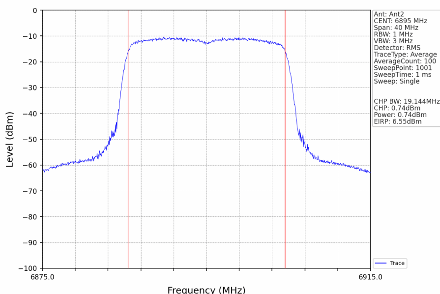
802.11ax(HEW20)_LCH_6895MHz_RU242_Left_Ant2_NTNV
