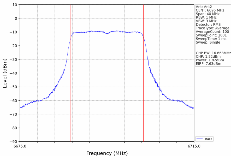
802.11a_MCH_6695MHz_Ant2_NTNV
