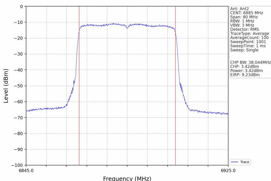
802.11ax(HEW40)_HCH_6885MHz_RU484_Left_Ant2_NTNV
