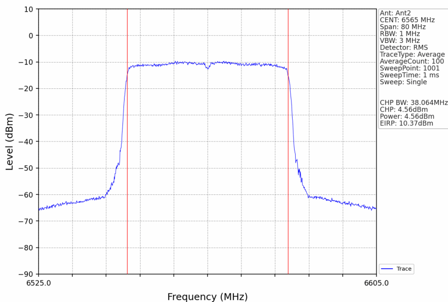
802.11ax(HEW40)_LCH_6565MHz_RU484_Left_Ant2_NTNV
