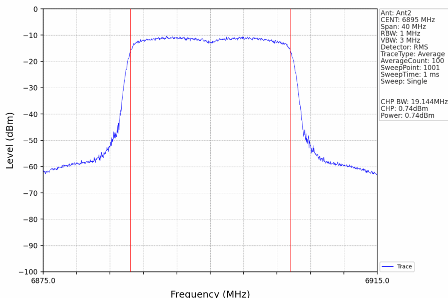
802.11ax(HEW20)_LCH_6895MHz_RU242_Left_Ant2_NTNV
