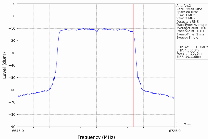
802.11ax(HEW40)_MCH_6685MHz_RU484_Left_Ant2_NTNV
