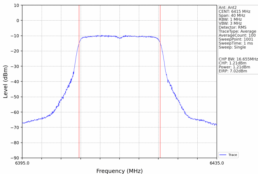
802.11a_HCH_6415MHz_Ant2_NTNV
