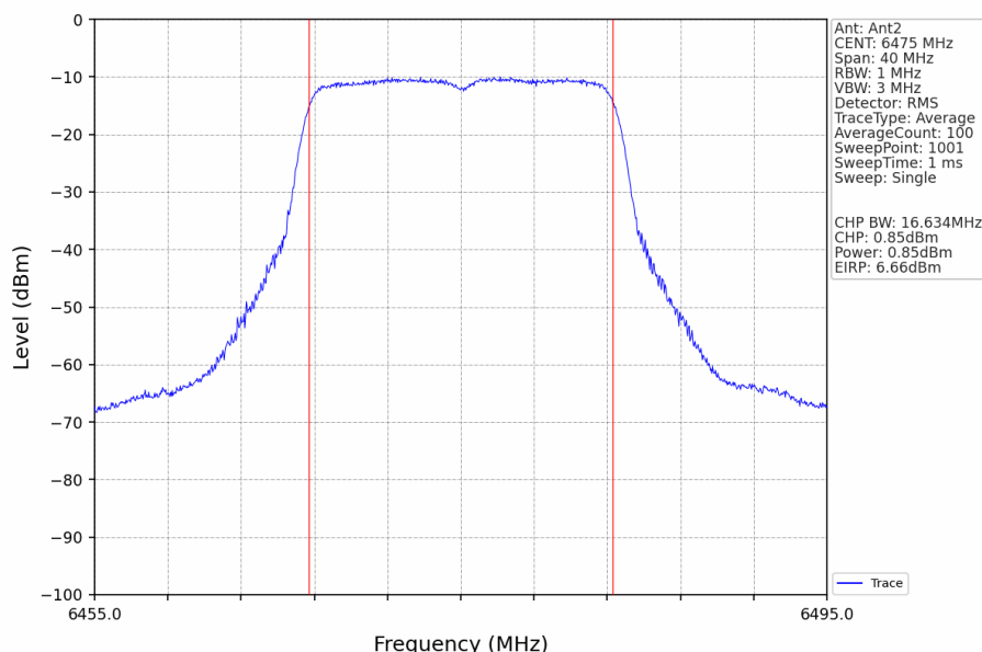
802.11a_MCH_6475MHz_Ant2_NTNV
