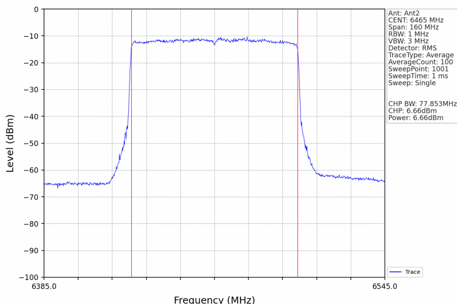
802.11ax(HEW80)_LCH_6465MHz_RU996_Left_Ant2_NTNV
