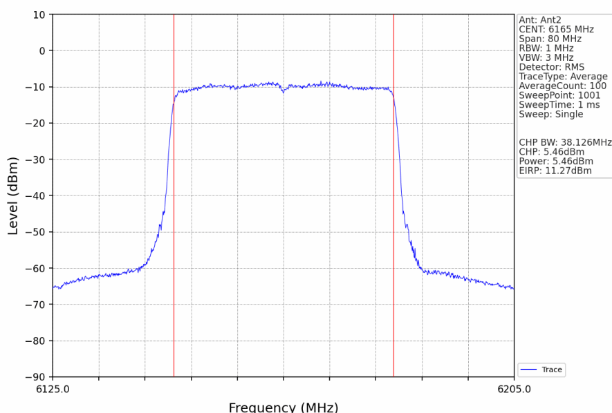
802.11ax(HEW40)_MCH_6165MHz_RU484_Left_Ant2_NTNV
