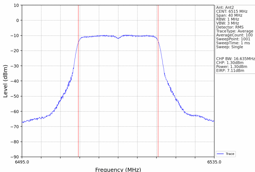
802.11a_HCH_6515MHz_Ant2_NTNV
