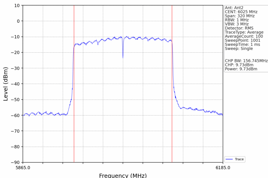
802.11ax(HEW160)_LCH_6025MHz_2xRU996_Left_Ant2_NTNV
