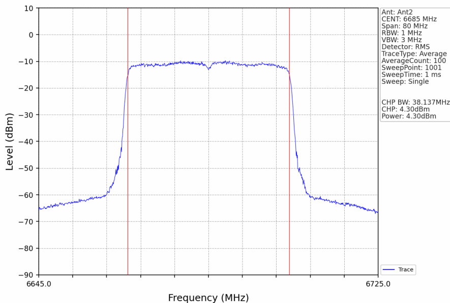
802.11ax(HEW40)_MCH_6685MHz_RU484_Left_Ant2_NTNV
