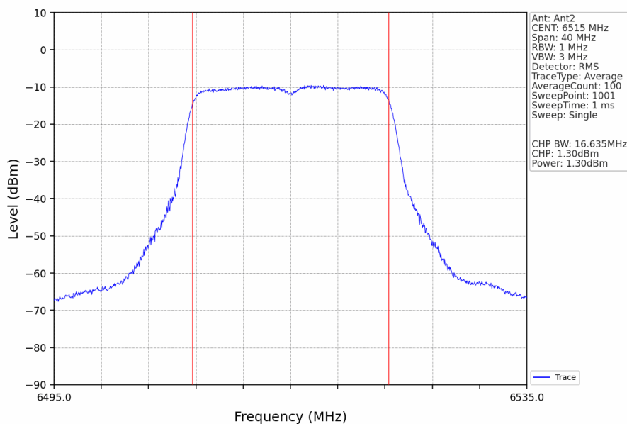
802.11a_HCH_6515MHz_Ant2_NTNV
