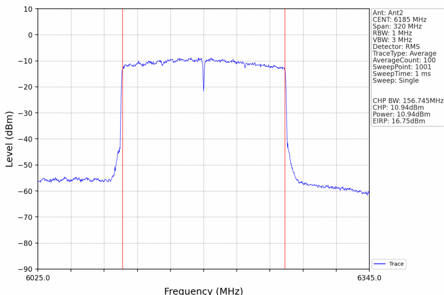
802.11ax(HEW160)_MCH_6185MHz_2xRU996_Left_Ant2_NTNV
