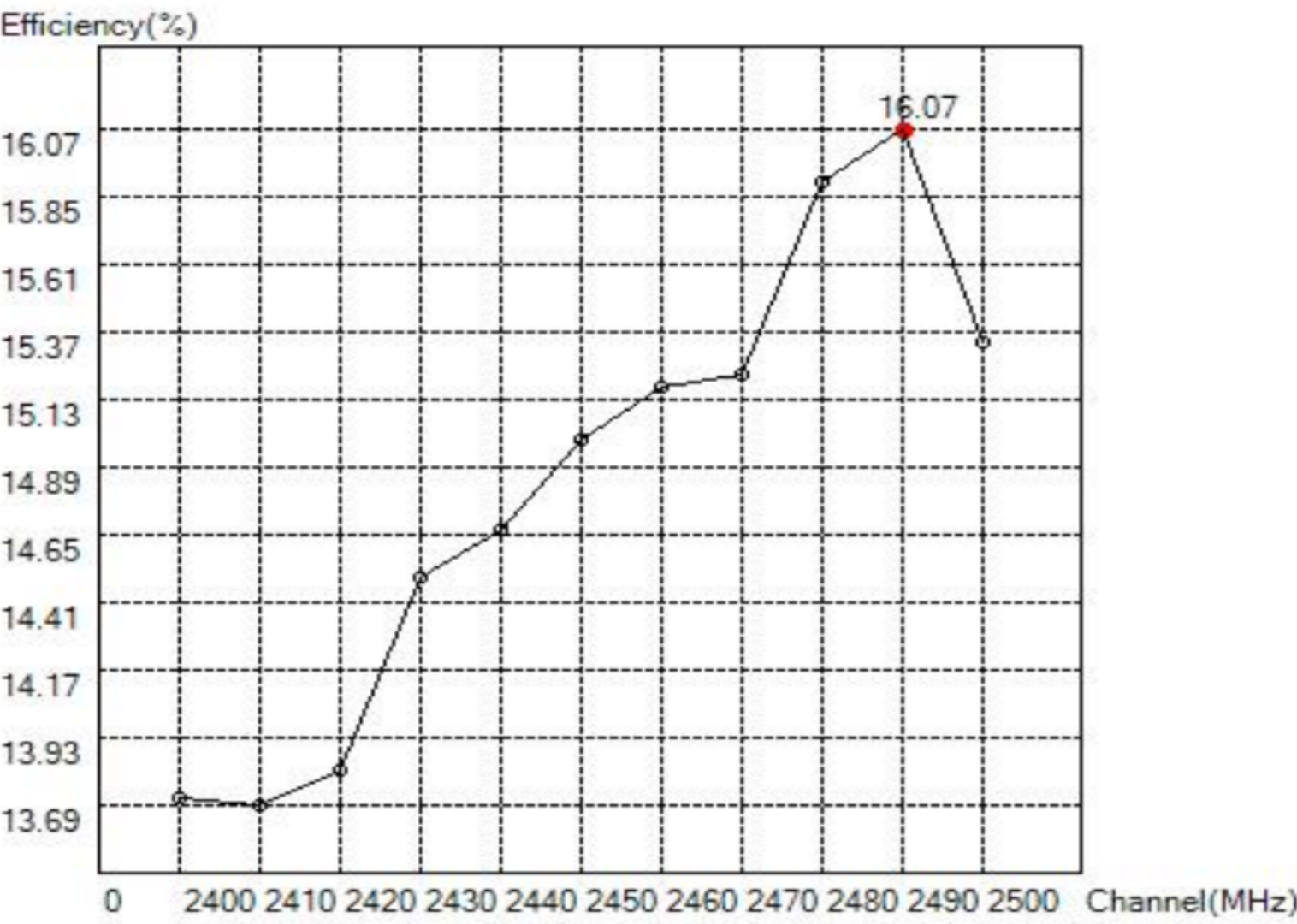
Efficiency-Plane
