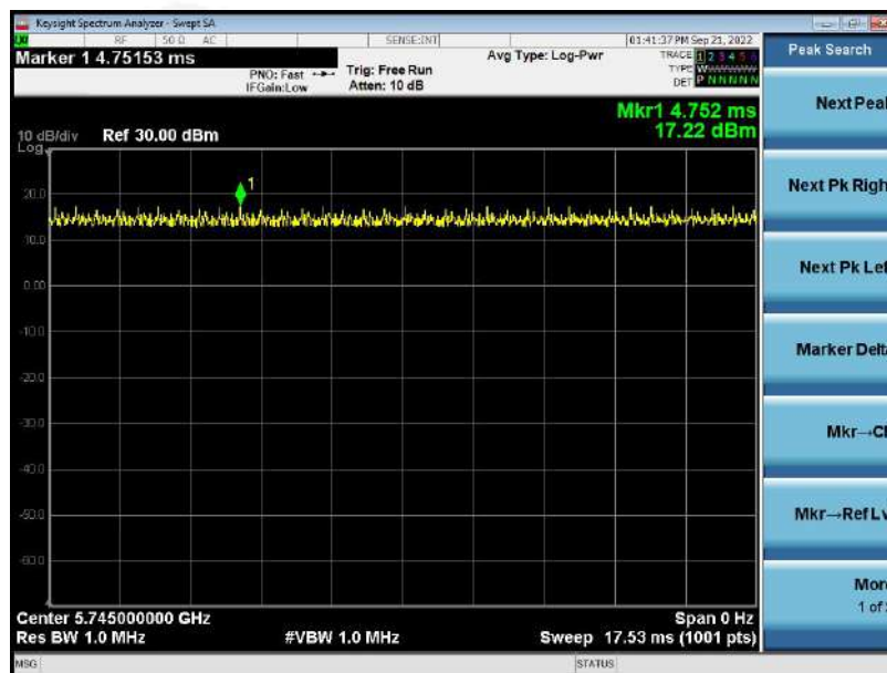
802.11 a CH149
