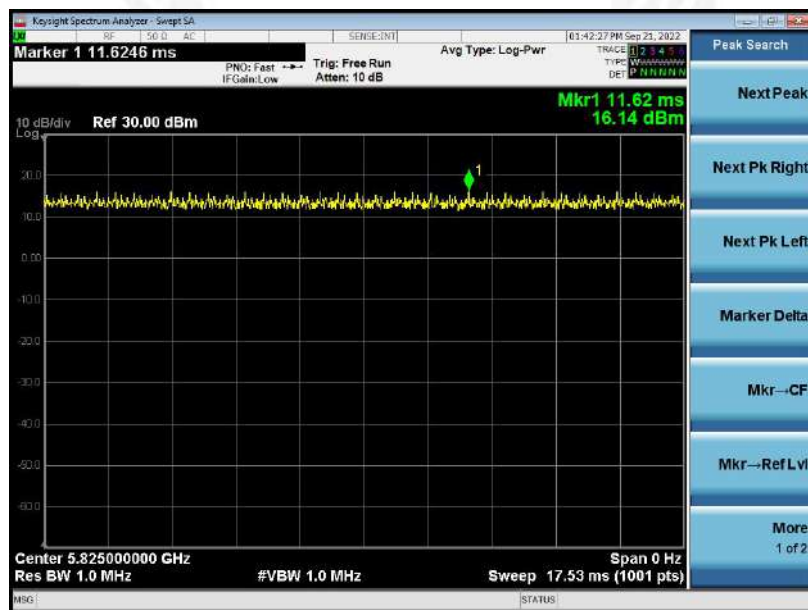
802.11 a CH165
