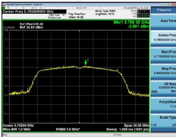
5785MHz
