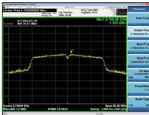
ANT2- 802.11ax HE40
