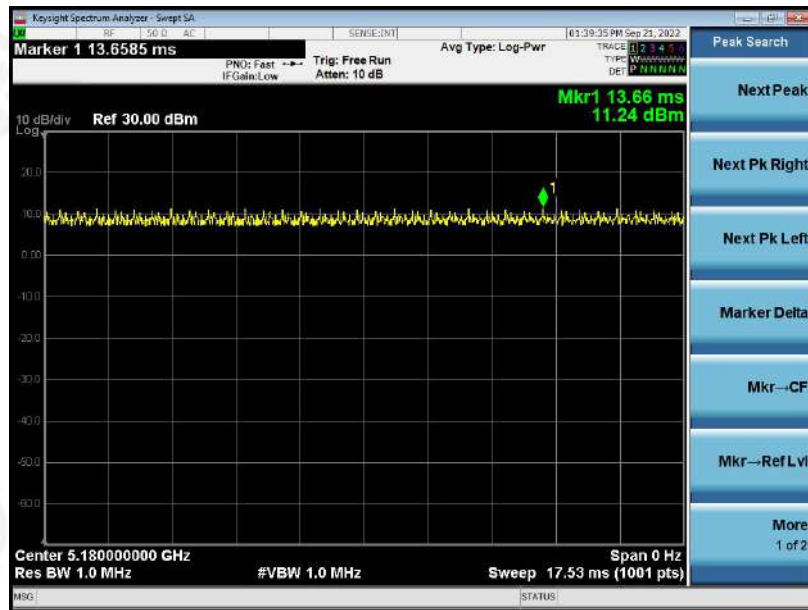
802.11 a CH36
