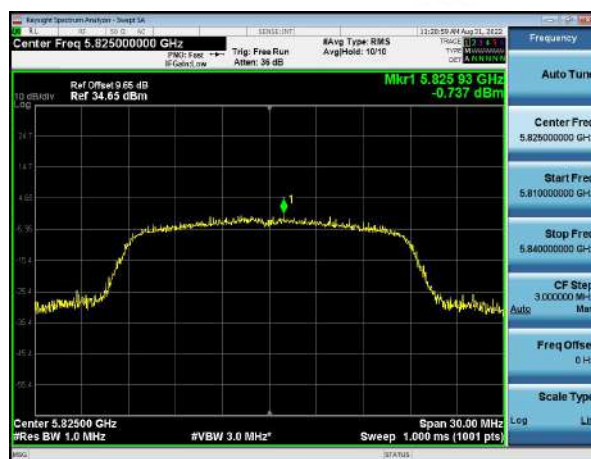
5825MHz
