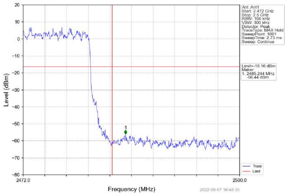
Pi/4DQPSK_2DH5_HOPP_Ant1_NTNV
