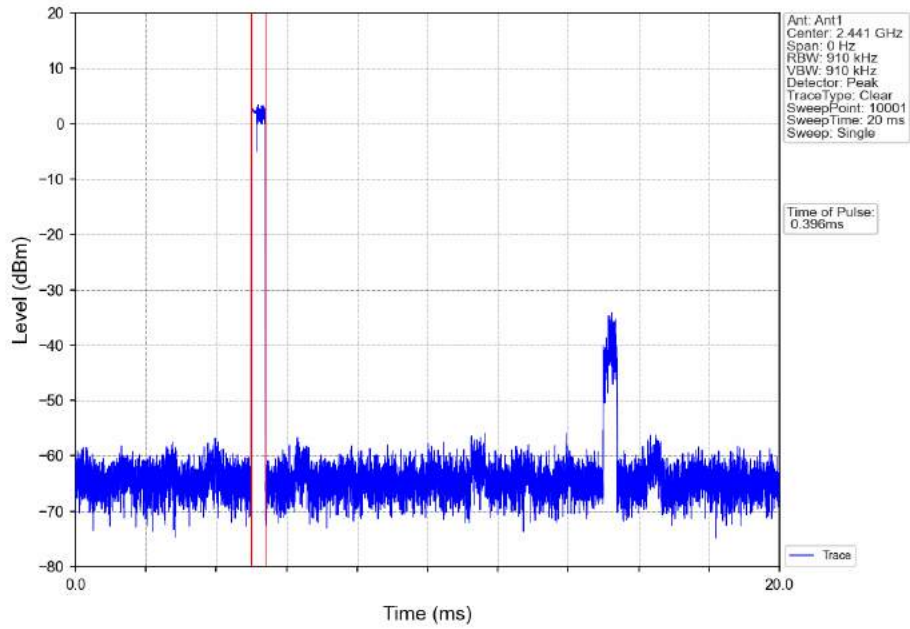
8DPSK_3DH1_HOPP_Ant1_NTNV
