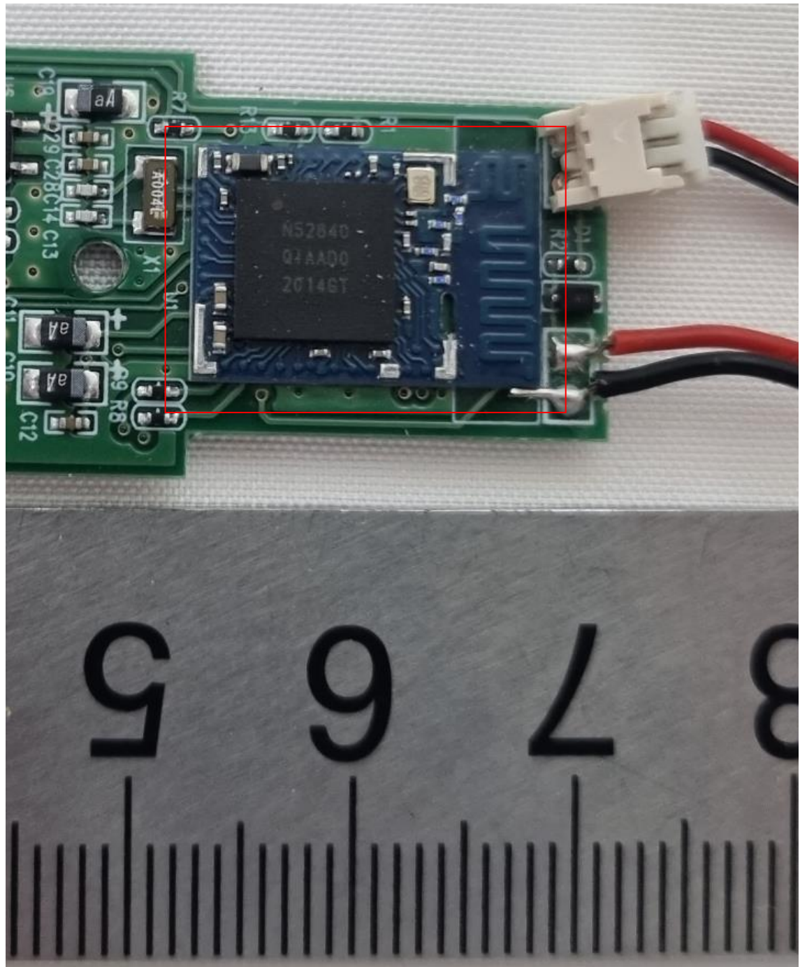
BT Module
