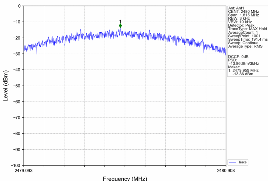
BLE_HCH_2480MHz_Ant1_NTNV
