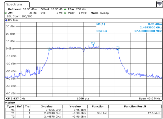
802.11n20_2437MHz
