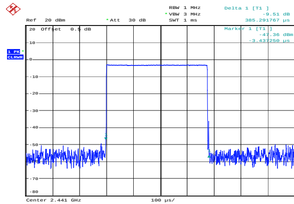
GFSK_Hopping_DH1 0.385ms
