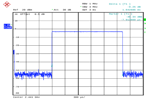
GFSK_Hopping_DH3 1.643ms
