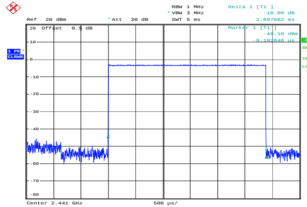
GFSK_Hopping_DH5 2.898ms
