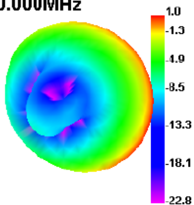
2450.000MHz
