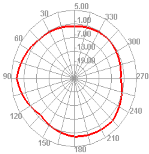
2500.000MHz H
