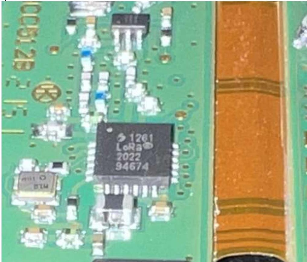
6) EUT Photo
