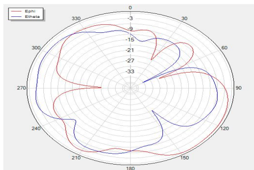
H Theta=90 freq=2400MHz
