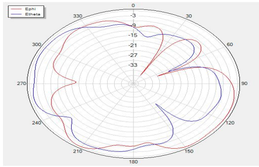
H Theta=90 freq=2420MHz
