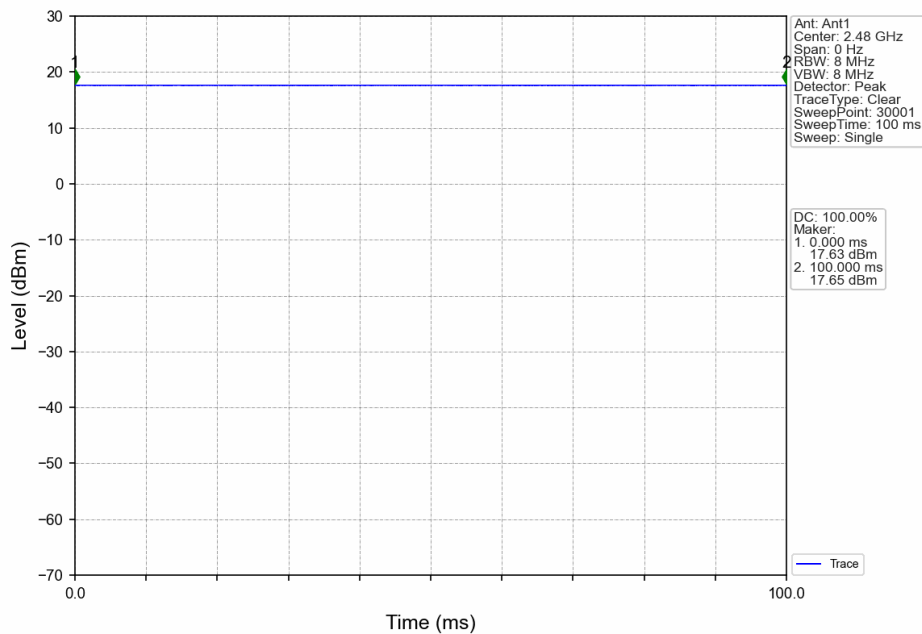
Zigbee_HCH_2480MHz_Ant1_NTNV
