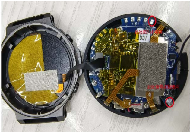
馈地处贴弹片，GND处贴1pF电容
