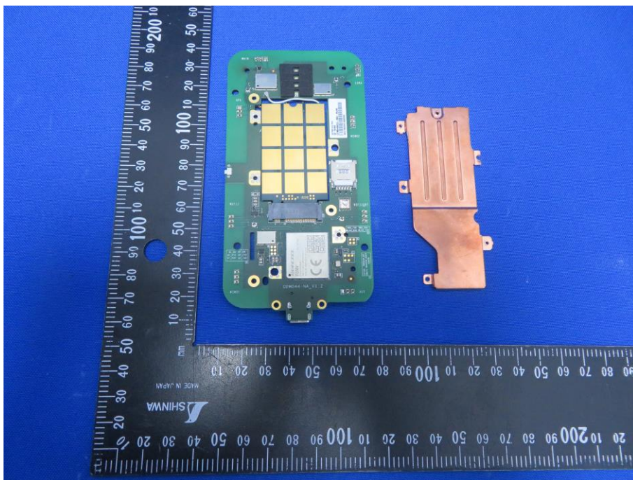
(12) EUT Photo
