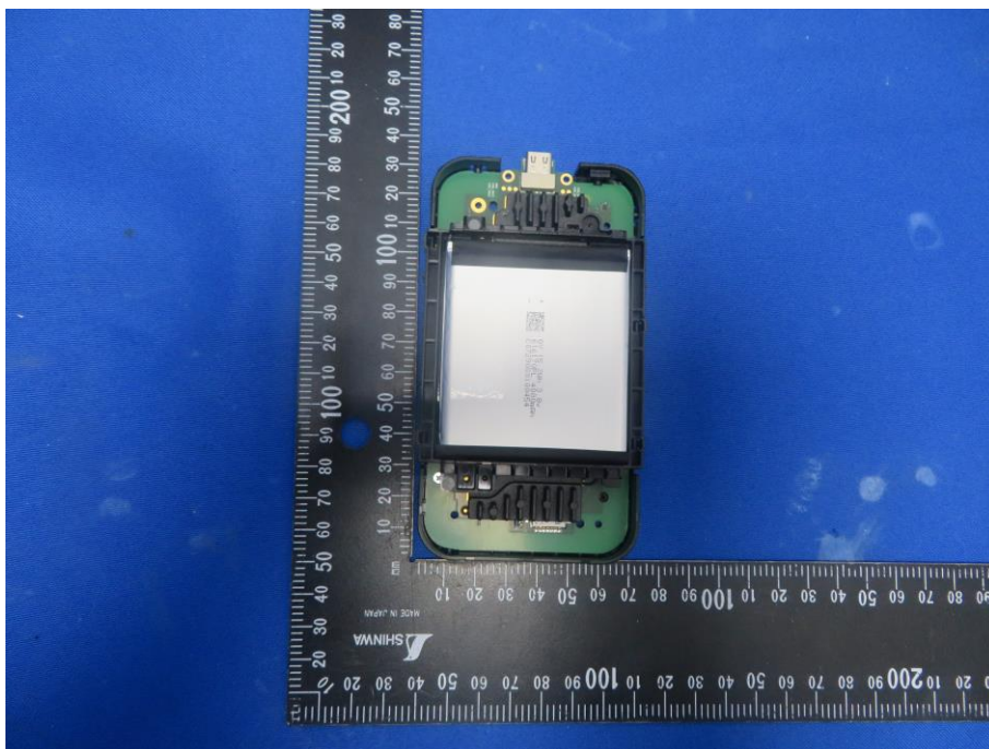
(4) EUT Photo
