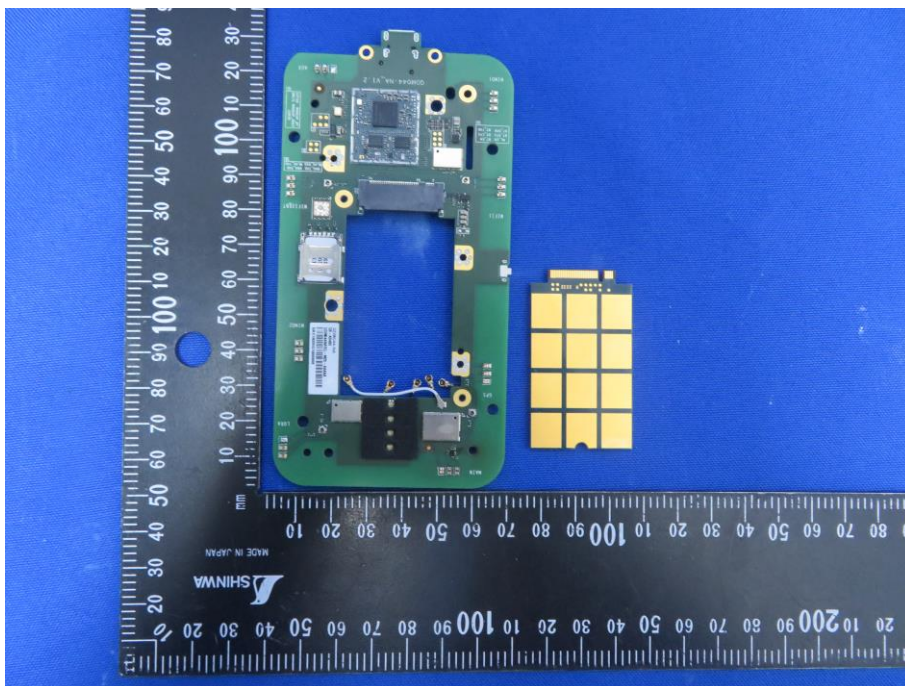
(14) EUT Photo
