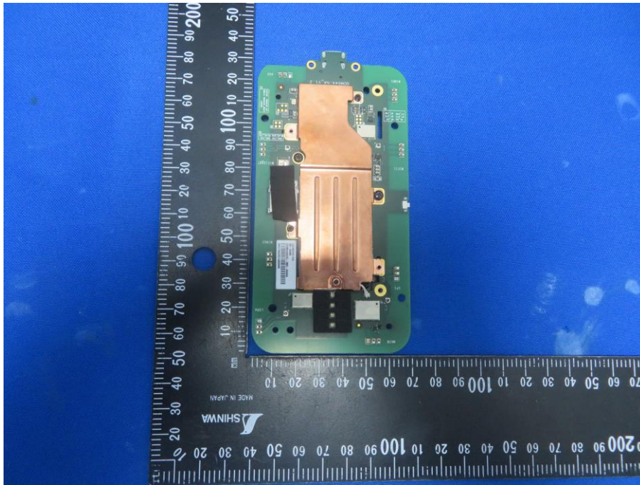
(9) EUT Photo
