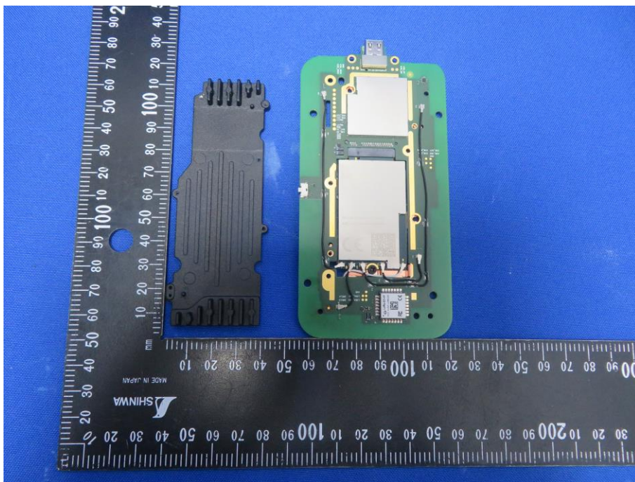
(10) EUT Photo
