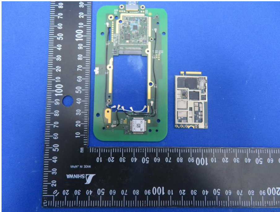
(13) EUT Photo
