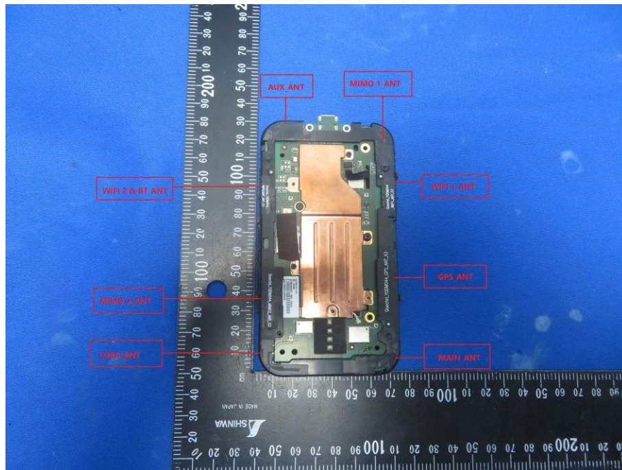
(5) EUT Photo
