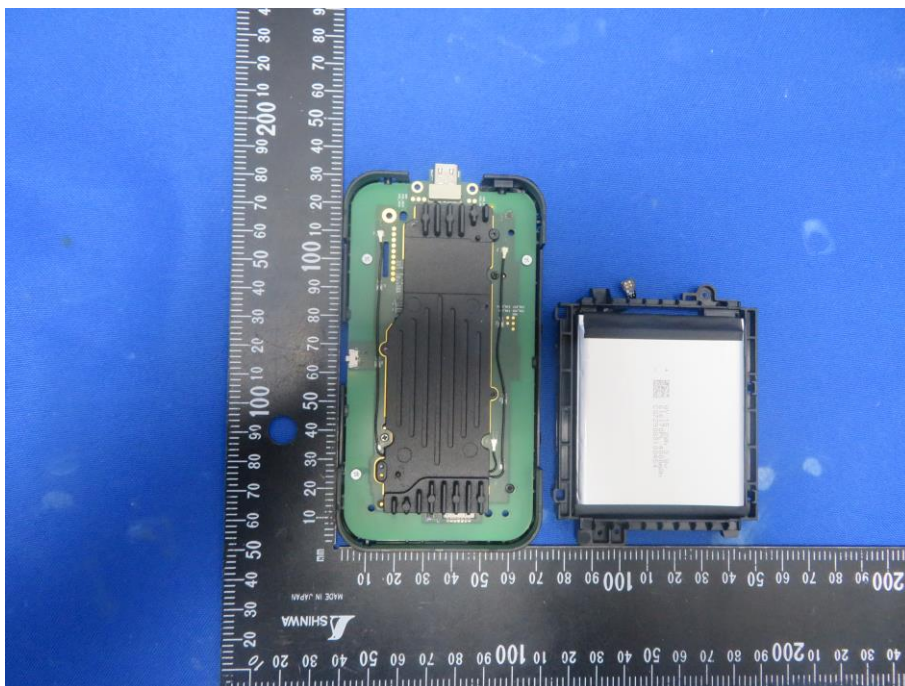
(6) EUT Photo
