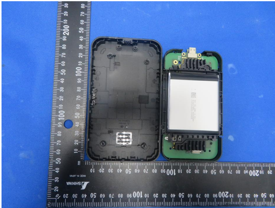
(3) EUT Photo
