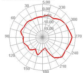
5850.000MHz E2
