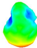
5850.000MHz E1
