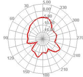
5850.000MHz E1
