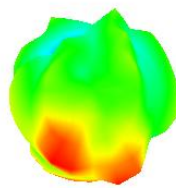
2450.000MHz E1
