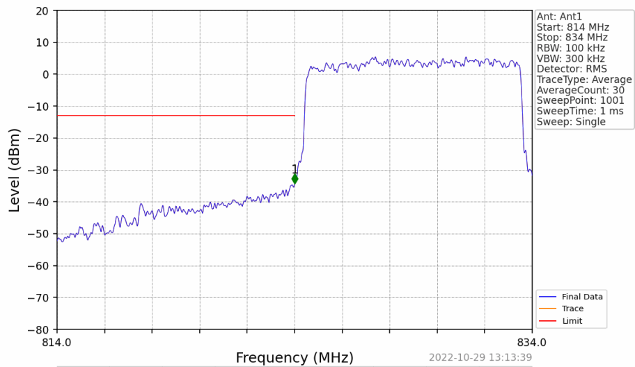
Band5_10MHz_QPSK_LCH_829MHz_RB_50_0_NTNV
