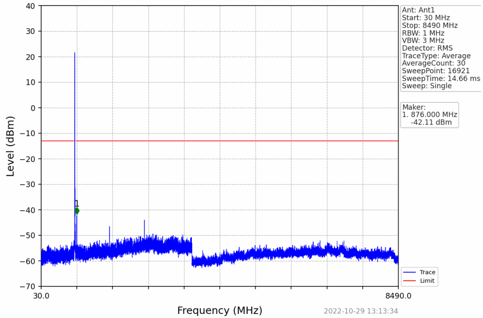
Band5_10MHz_QPSK_LCH_829MHz_RB_50_0_NTNV
