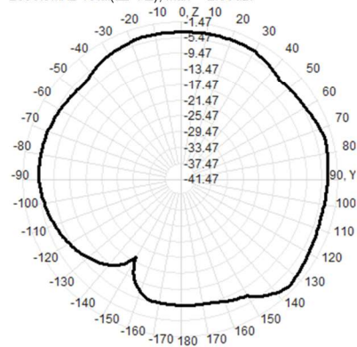
2500.0MHz Total(E2-YZ), Max= -2.95dBi
