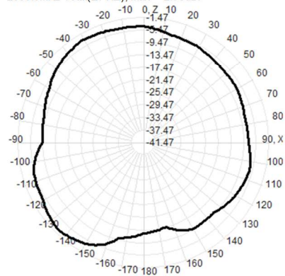
2500.0MHz Total(E1-XZ), Max= -2.78dBi
