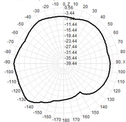
2450.0MHz Total(E1-XZ), Max= -2.52dBi
