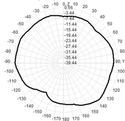
2450.0MHz Total(E2-YZ), Max= -2.42dBi
