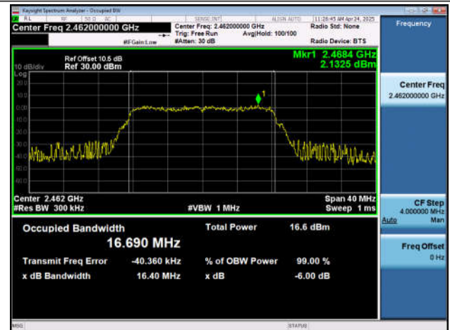
11G-Ant1-2462
