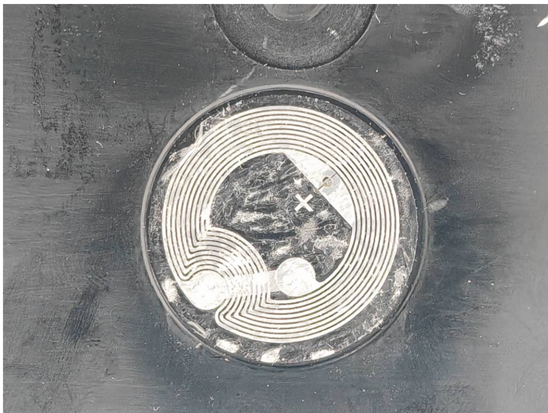
NFC Tag
