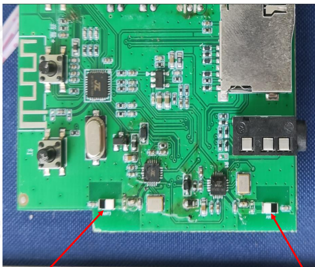
Antenna2
