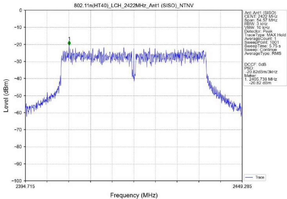
802.11n(HT40)_LCH_2422MHz_Ant1 (SISO)_NTNV
