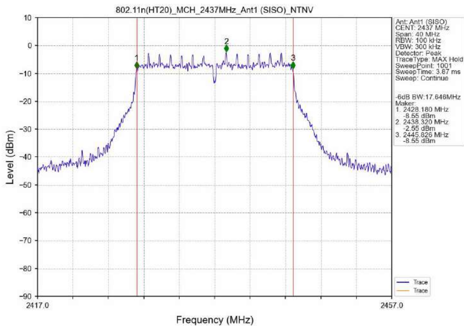
802.11n(HT20)_MCH_2437MHz_Ant1 (SISO)_NTNV
