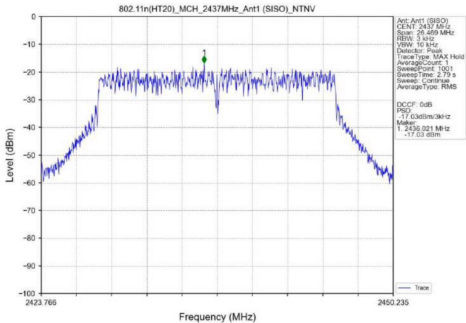
802.11n(HT20)_MCH_2437MHz_Ant1 (SISO)_NTNV
