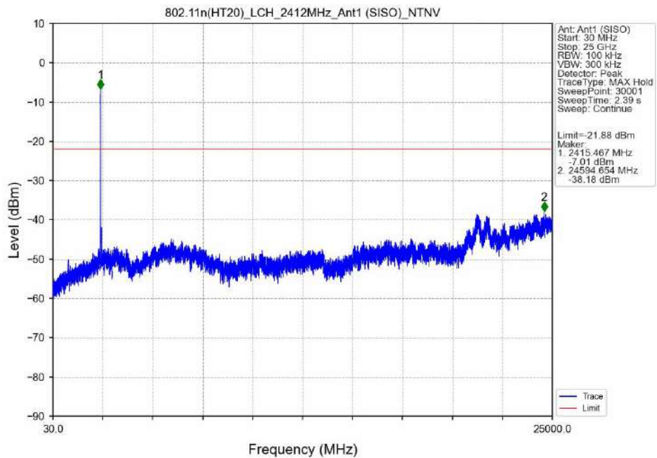
802.11n(HT20)_LCH_2412MHz_Ant1 (SISO)_NTNV
