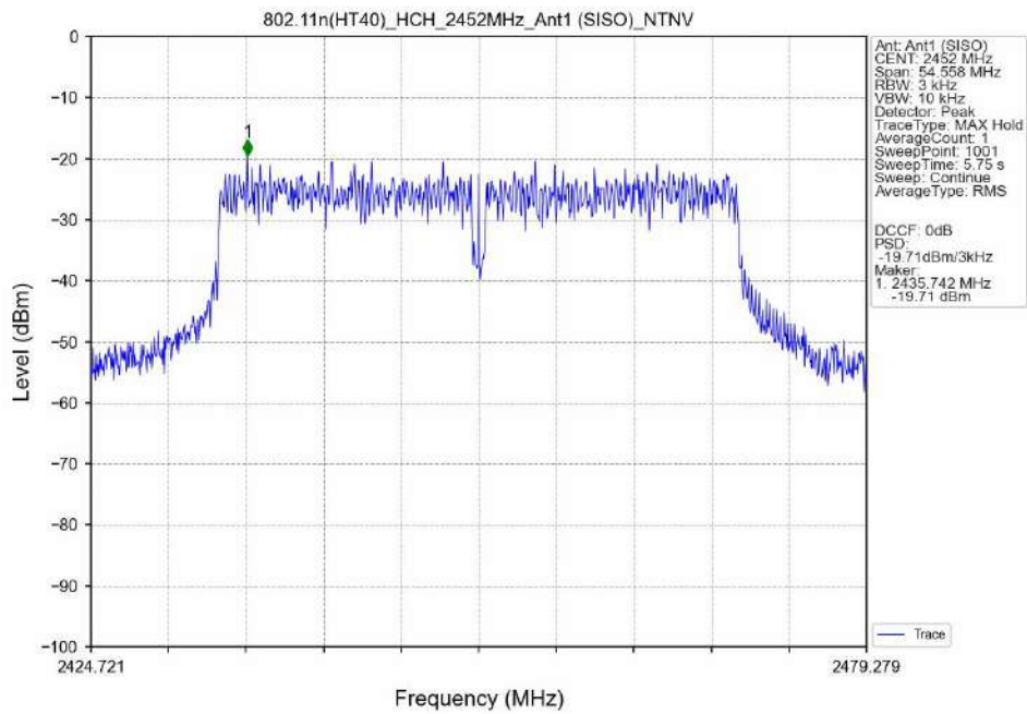
802.11n(HT40)_HCH_2452MHz_Ant1 (SISO)_NTNV
