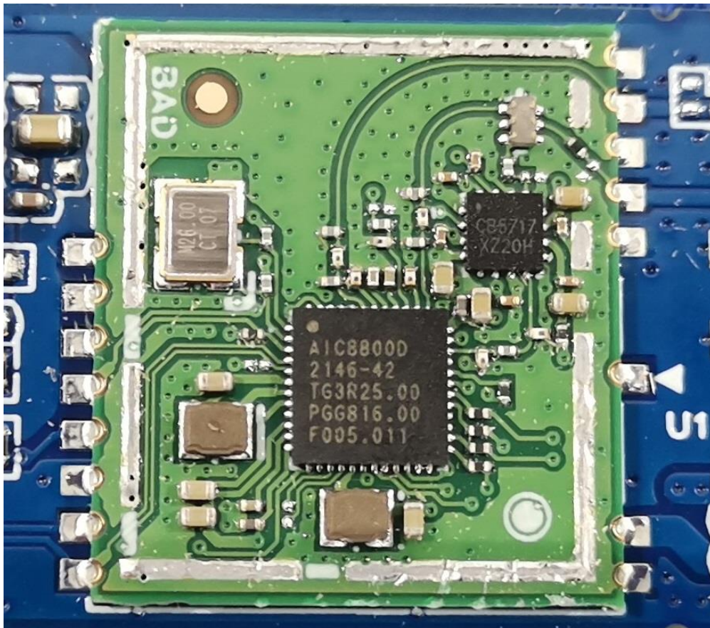
4) EUT Photo
