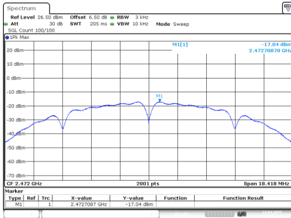
802.11b_2472MHz
