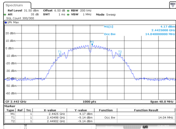
802.11b_2442MHz
