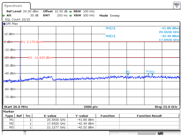
802.11b_2442MHz
