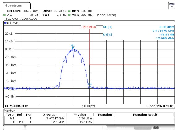
802.11b_2472MHz
