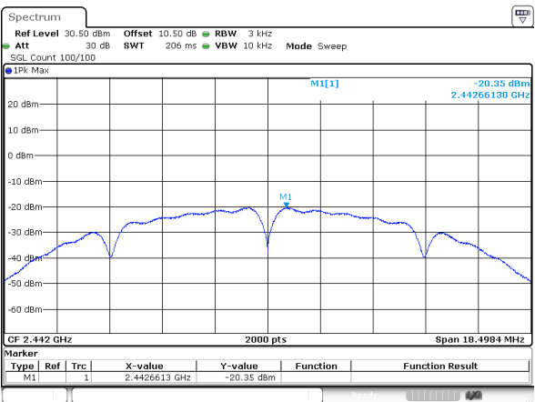
802.11b_2442MHz
