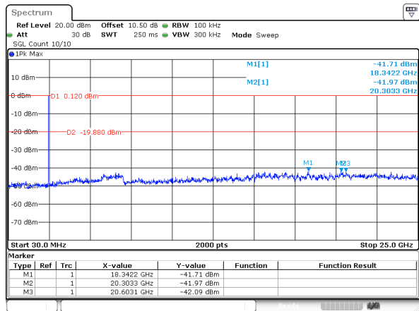
802.11b_2472MHz
