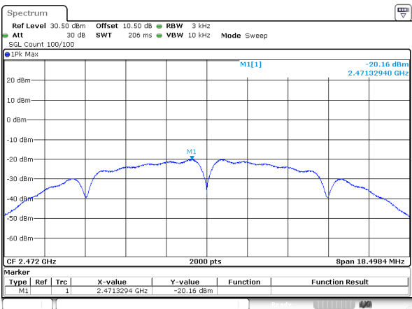
802.11b_2472MHz
