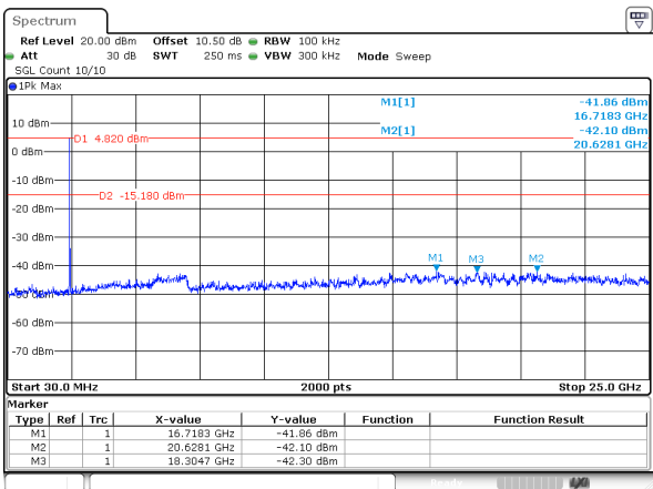
802.11b_2442MHz
