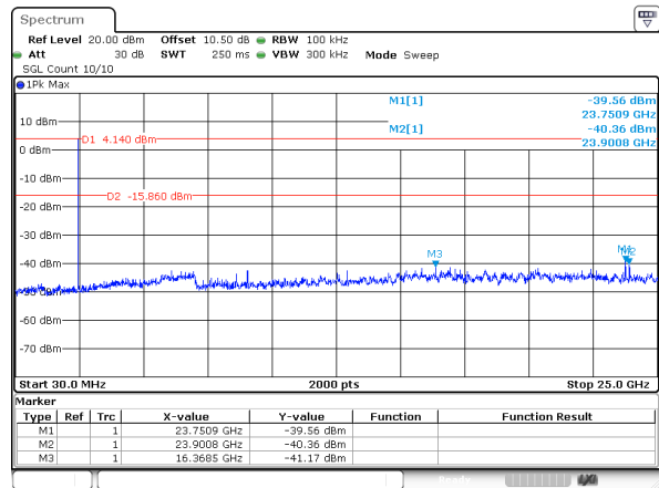
802.11b_2472MHz
